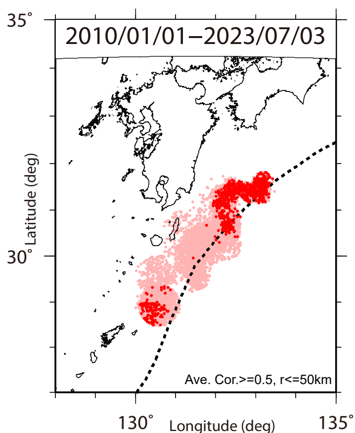
第1図. 2010年1月1日から2023年7月3日までの期間内に波形相関解析 [Asano et al. (2015)] によって検出された超低周波イベントの震央分布. 検出イベントを防災科研 Hi-net の手動または自動検測震源と照合して通常の地震を除去した後、それ以外を超低周波イベントとして桃色（2023年3月31日以前）、および赤色（4月1日以降）の点でそれぞれ示す。
