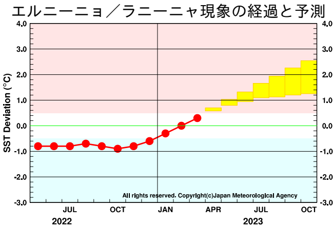
図 1 エルニーニョ監視海域の海面水温の基準値との差の 5 か月移動平均値 3 月までの経過（観測値）を折れ線グラフで、大気海洋結合モデルによる予測結果（70%の確率で入ると予想される範囲）をボックスで示している。指数が赤／青の範囲に入っている期間がエルニーニョ／ラニーニャ現象の発生期間である。エルニーニョ監視海域の海面水温の基準値はその年の前年までの 30 年間の各月の平均値。
