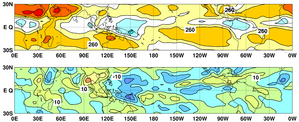
図 9 外向き長波放射量 (OLR) (上) 及び年偏差 (下) の分布図 (2023 年 5 月)
