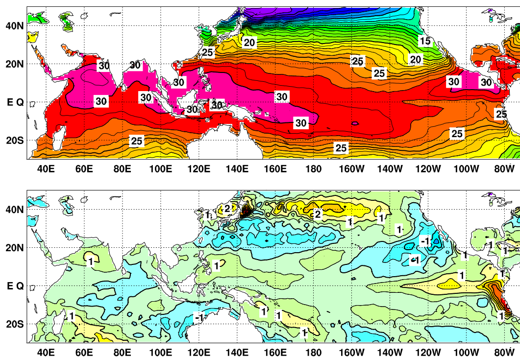
図4 2023年5月の海面水温図（上）及び平年偏差図（下）
