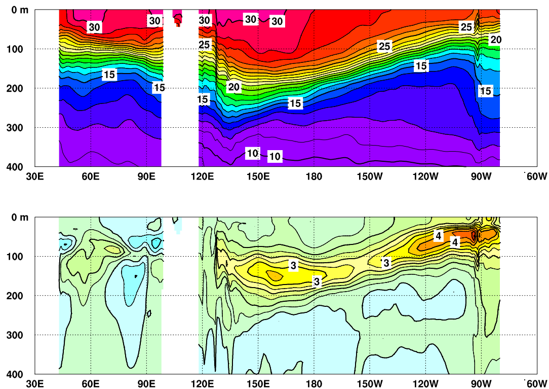
図5 2023年5月のインド洋から太平洋の赤道に沿った水温（上）及び平年偏差（下）の断面図
