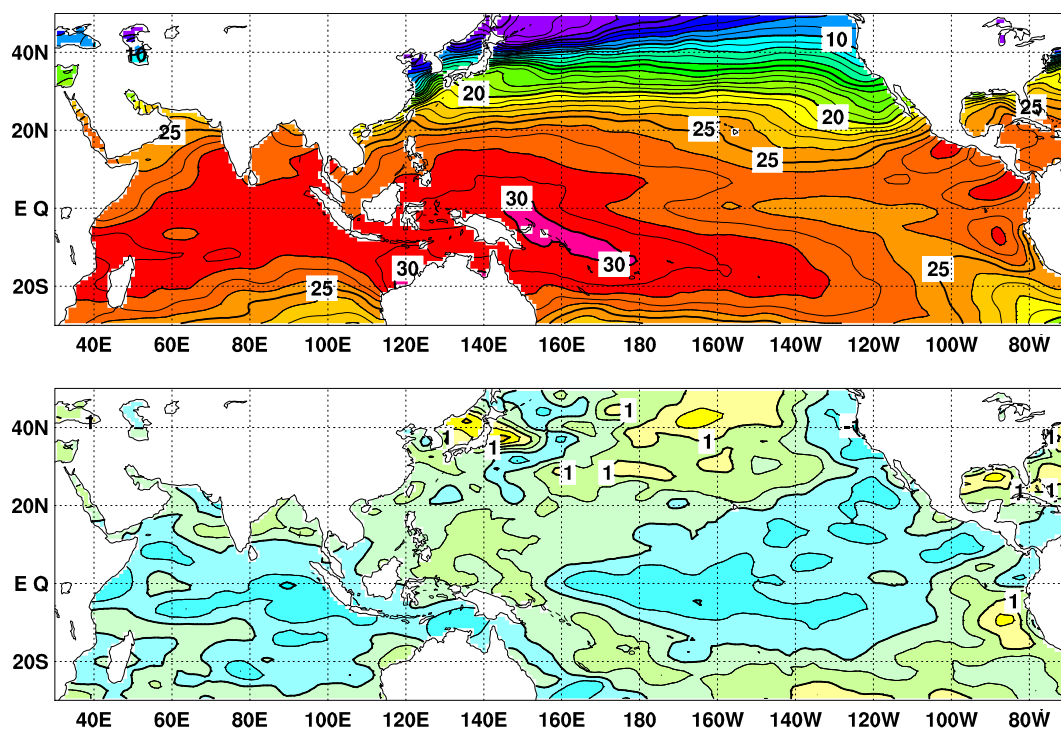
図4 2023年2月の海面水温図(上)及び平年偏差図(下)
