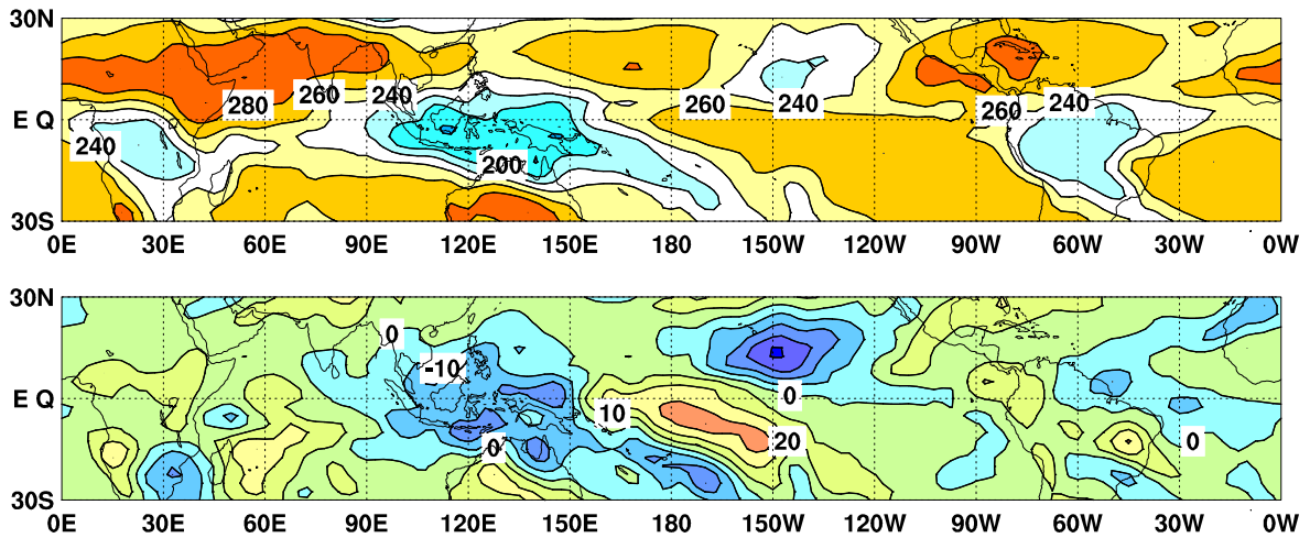
図9 外向き長波放射量 (OLR) (上) 及び年偏差 (下) の分布図 (2023年2月)
