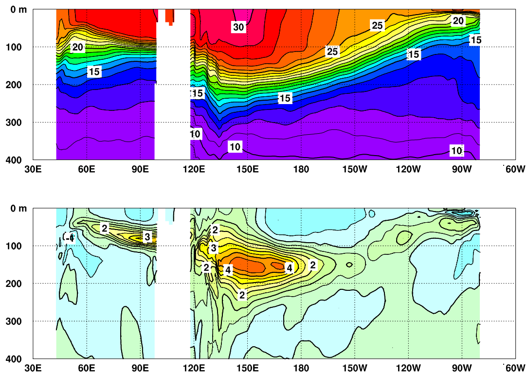
図5 2023年2月のインド洋から太平洋の赤道に沿った水温(上)及び平年偏差(下)の断面図
