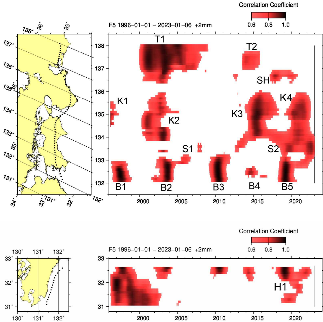
第1図 長期的スロースリップ客観検知図（1996年から2023年1月）
