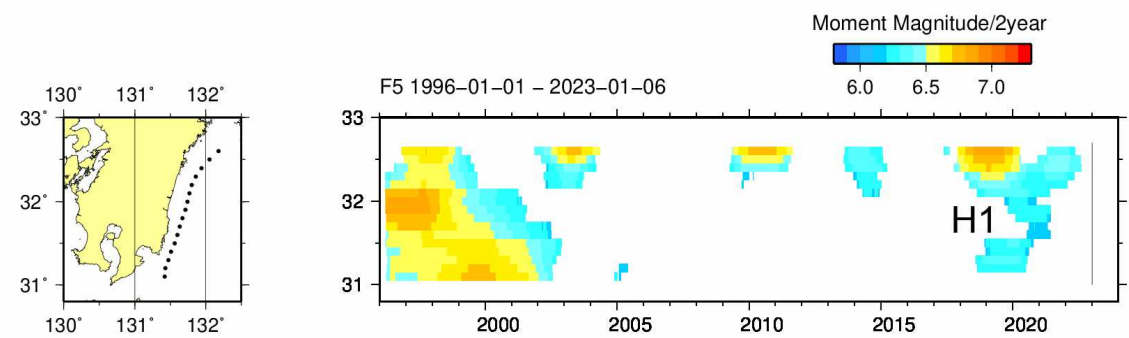
第2図 長期的スロースリップの規模分布（1996年から2023年1月） 2年間あたりの変化量から推定したモーメントマグニチュード。地域略号は第1図と同じ。
