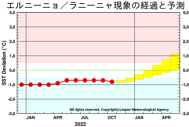
図 1 エルニーニョ監視海域の海面水温の基準値との差の 5 か月移動平均値 10 月までの経過（観測値）を折れ線グラフで、大気海洋結合モデルによる予測結果（70%の確率で入ると予想される範囲）をボックスで示している。指数が赤／青の範囲に入っている期間がエルニーニョ／ラニーニャ現象の発生期間である。エルニーニョ監視海域の海面水温の基準値はその年の前年までの 30 年間の各月の平均値。
