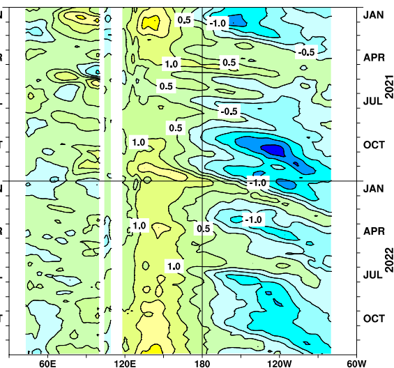
図 7 インド洋から太平洋の赤道に沿った海面から深度 300m までの平均水温平年偏差の経度-時間断面図
