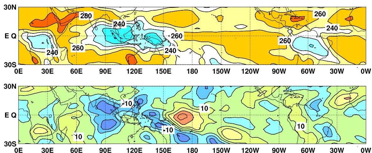
図 9 外向き長波放射量 (OLR) (上) 及び年偏差 (下) の分布図 (2022 年 12 月)
