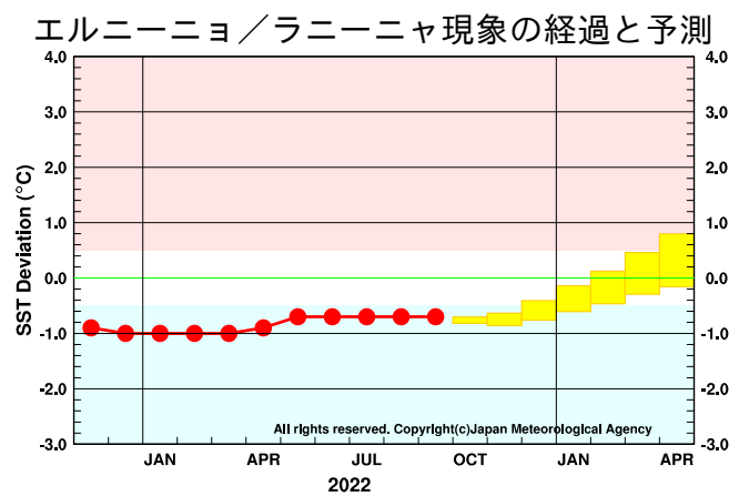
図 1 エルニーニョ監視海域の海面水温の基準値との差の 5 か月移動平均値 9 月までの経過（観測値）を折れ線グラフで、大気海洋結合モデルによる予測結果（70%の確率で入ると予想される範囲）をボックスで示している。指数が赤／青の範囲に入っている期間がエルニーニョ／ラニーニャ現象の発生期間である。エルニーニョ監視海域の海面水温の基準値はその年の前年までの 30 年間の各月の平均値。
