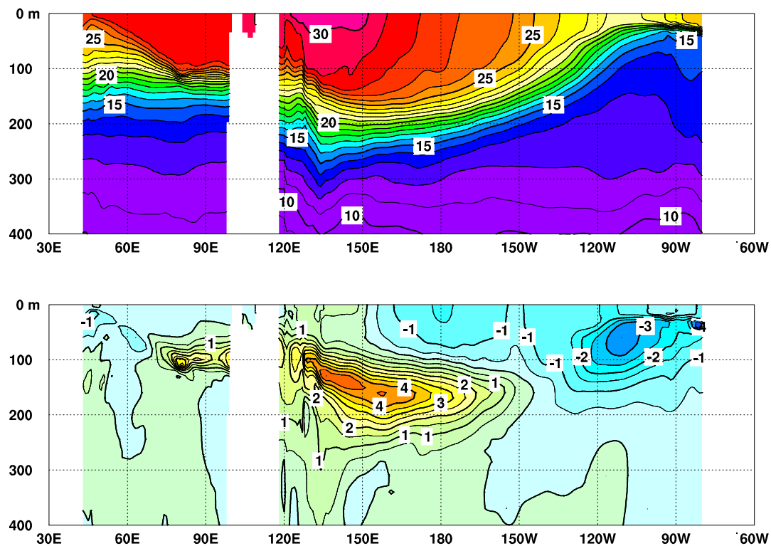
図5 2022年11月のインド洋から太平洋の赤道に沿った水温（上）及び平年偏差（下）の断面図
