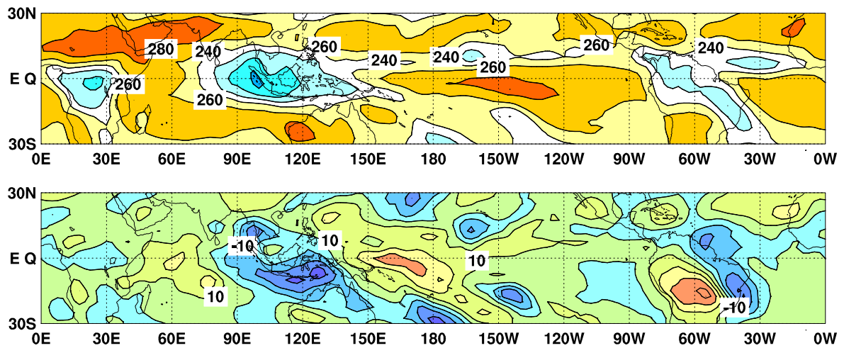
図 9 外向き長波放射量 (OLR) (上) 及び年偏差 (下) の分布図 (2022 年 11 月)
