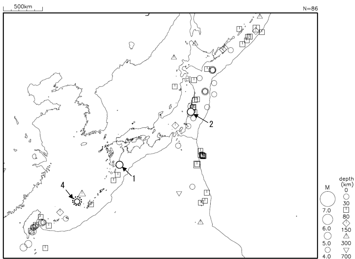
令和4年10月に発生したM4.0以上の地震（図中の番号は、表の番号に対応）
