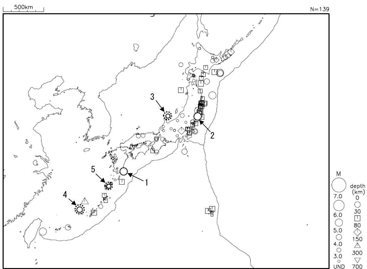
令和4年10月に震度1以上を観測した地震（図中の番号は、表の番号に対応）
