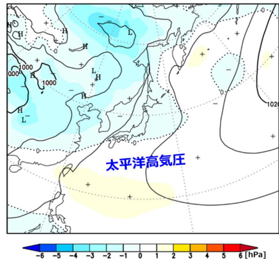
図6 2022年6～8月の3か月平均海面気圧（等値線）および平年偏差（陰影） 等値線間隔は4hPa。平年値は1991～2020年の30年平均値。（この図は6月1日～8月30日までのデータで作成しています。）
