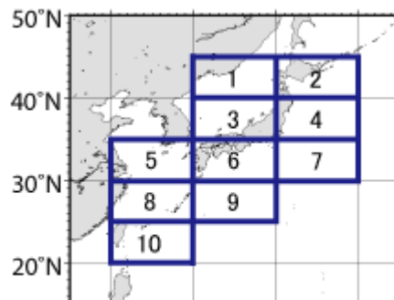
図 2 海面水温の海域区分
