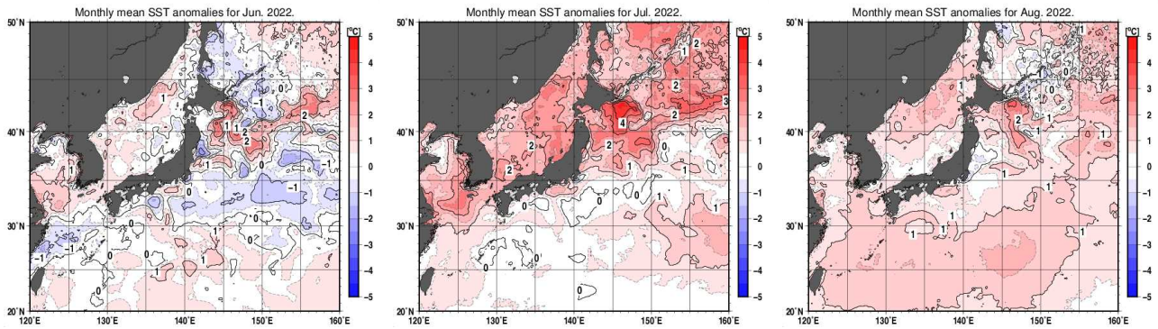
図5 2022年（令和4年）6月（左）、7月（中央）、8月（右）の日本近海の海面水温平年差図
