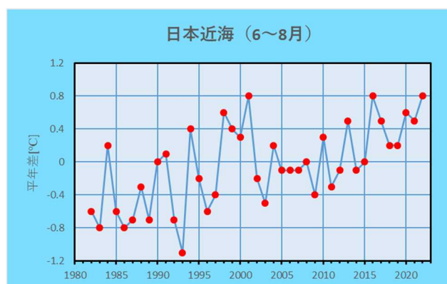
図 3 日本近海の 6～8 月の平均海面水温の平年差の経年変化
