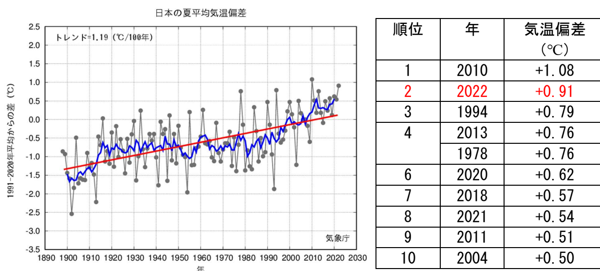
図1 日本の夏（6～8月）平均気温偏差の経年変化（1898～2022年）と順位表（上位10年） 折れ線グラフは各年の基準値からの偏差、青線は偏差の5年移動平均を、赤線は長期変化傾向を示す。基準値は1991～2020年の30年平均値。
