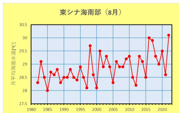
図 4 7 月の北海道南東方（海域 2）、8 月の東シナ海南部（海域 8）の月平均海面水温の推移（1982～2022 年）
