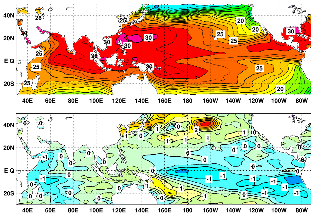
図4 2022年7月の海面水温図（上）及び平年偏差図（下）
