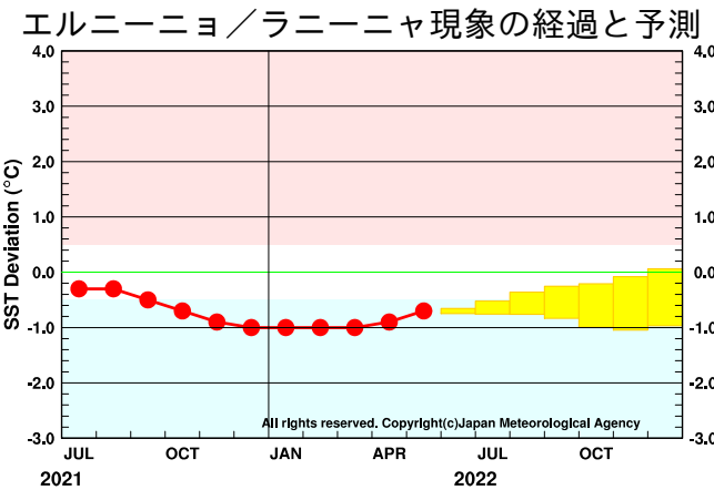
図 1 エルニーニョ監視海域の海面水温の基準値との差の 5 か月移動平均値 5 月までの経過（観測値）を折れ線グラフで、大気海洋結合モデルによる予測結果（70%の確率で入ると予想される範囲）をボックスで示している。指数が赤／青の範囲に入っている期間がエルニーニョ／ラニーニャ現象の発生期間である。エルニーニョ監視海域の海面水温の基準値はその年の前年までの 30 年間の各月の平均値。
