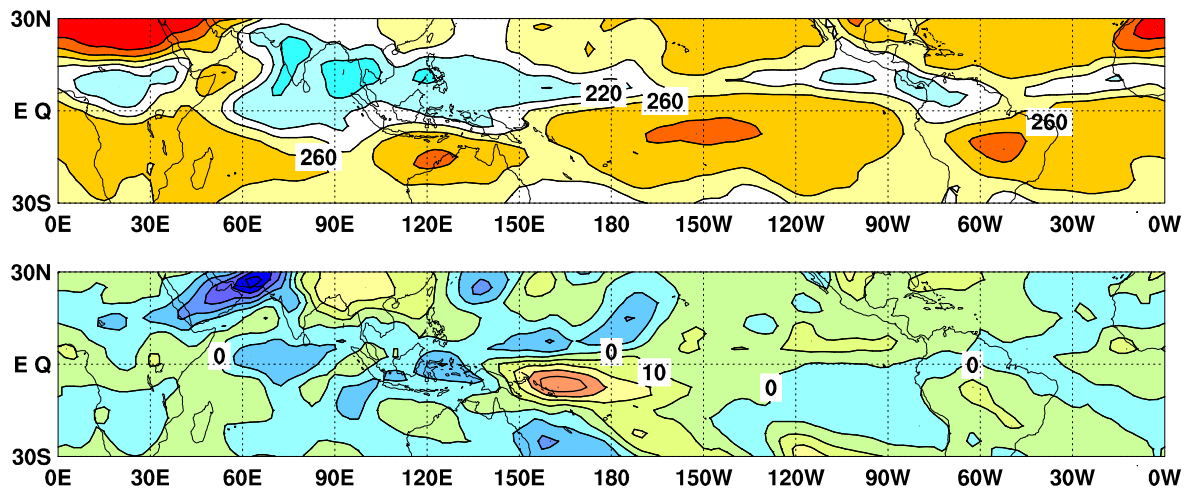
図 9 外向き長波放射量 (OLR) (上) 及び年々偏差 (下) の分布図 (2022 年 7 月)
