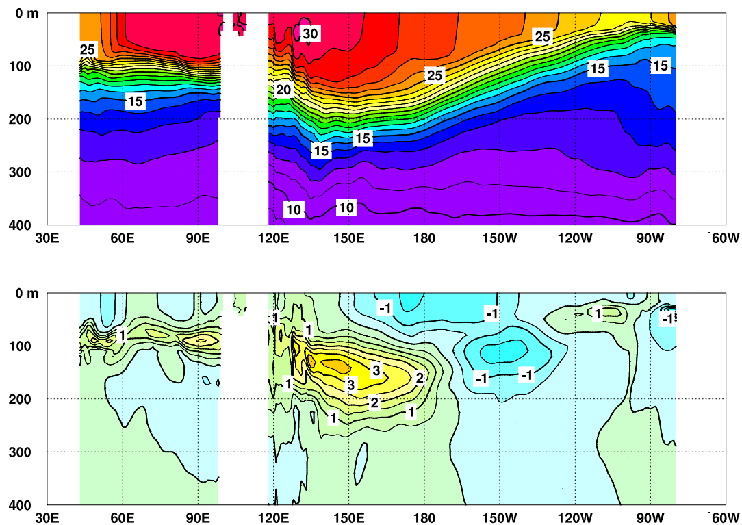
図5 2022年7月のインド洋から太平洋の赤道に沿った水温（上）及び平年偏差（下）の断面図
