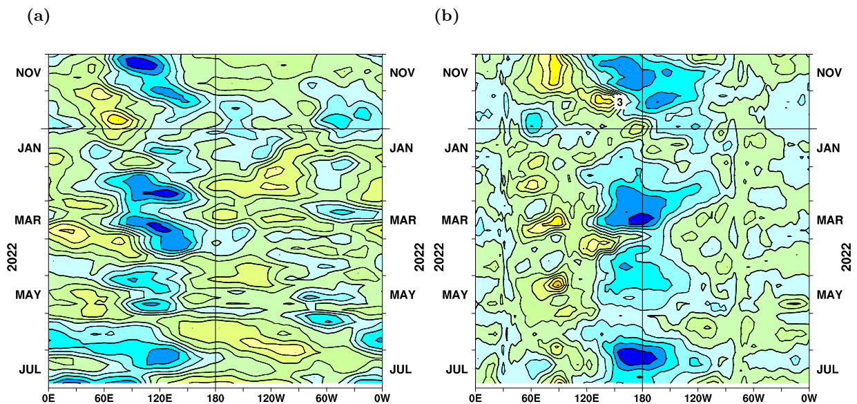
図 10 赤道付近における対流圏上層 (200hPa) の速度ポテンシャルの年々偏差 (a) 及び対流圏下層 (850hPa) の東西風速の年々偏差 (b) の経度-時間断面図
