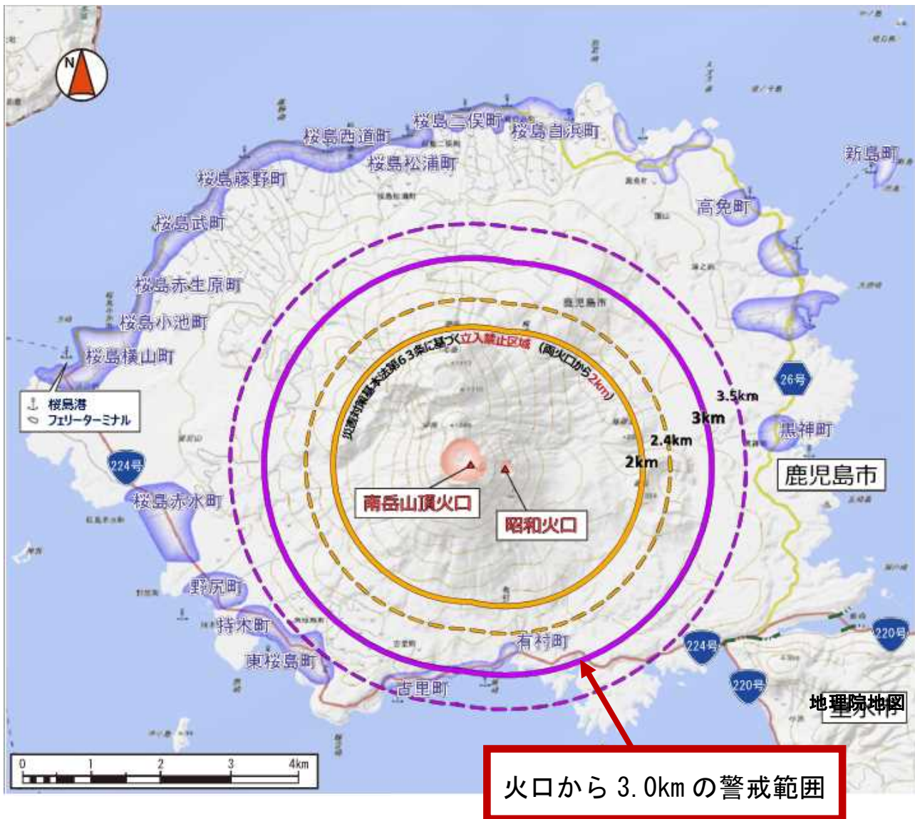
図1 桜島 警戒が必要な範囲
