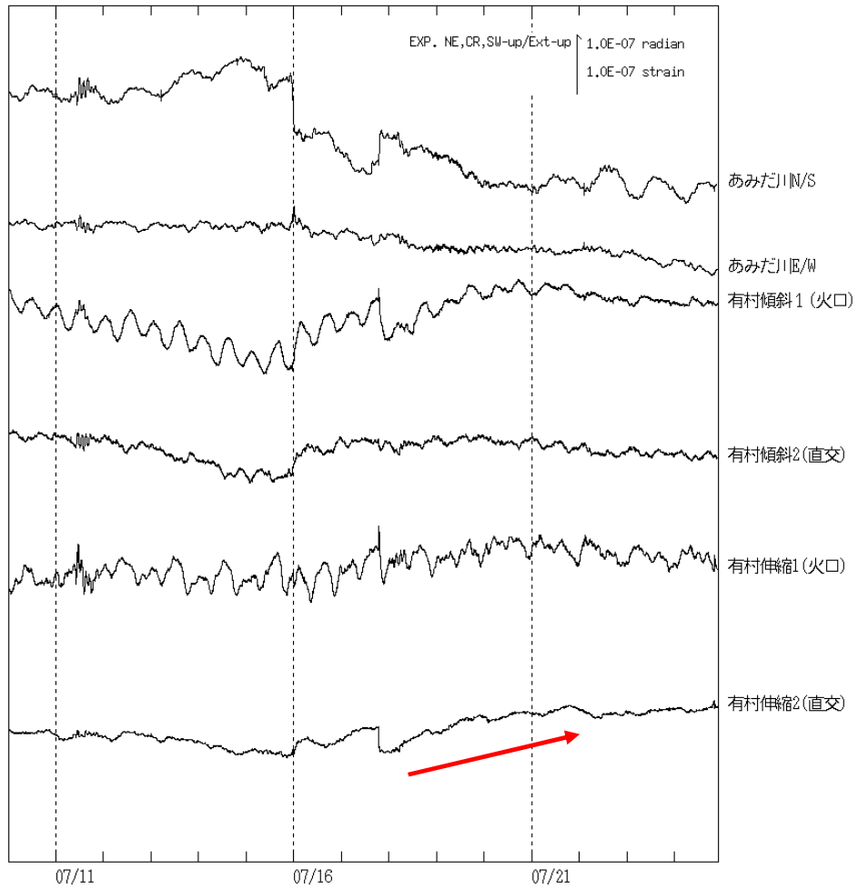
図3 桜島 伸縮計による地殻変動の状況 (有村坑道観測点(大隅河川国道事務所設置))
