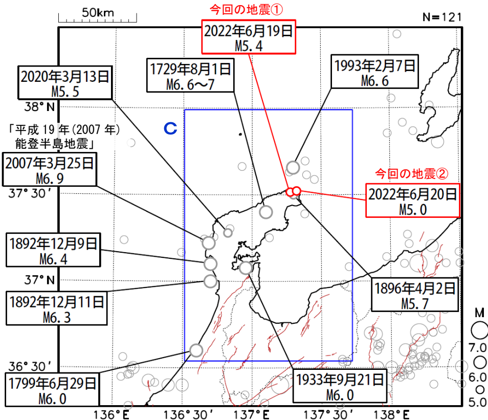
図2-8 震央分布図
