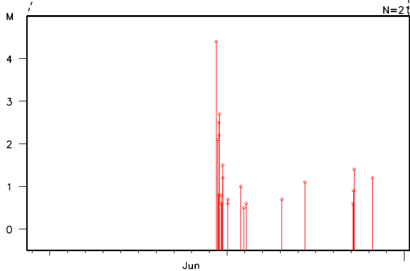
領域 a 内の M-T 図 6 月 10 日～6 月 30 日、 M \geq 0.5 )
