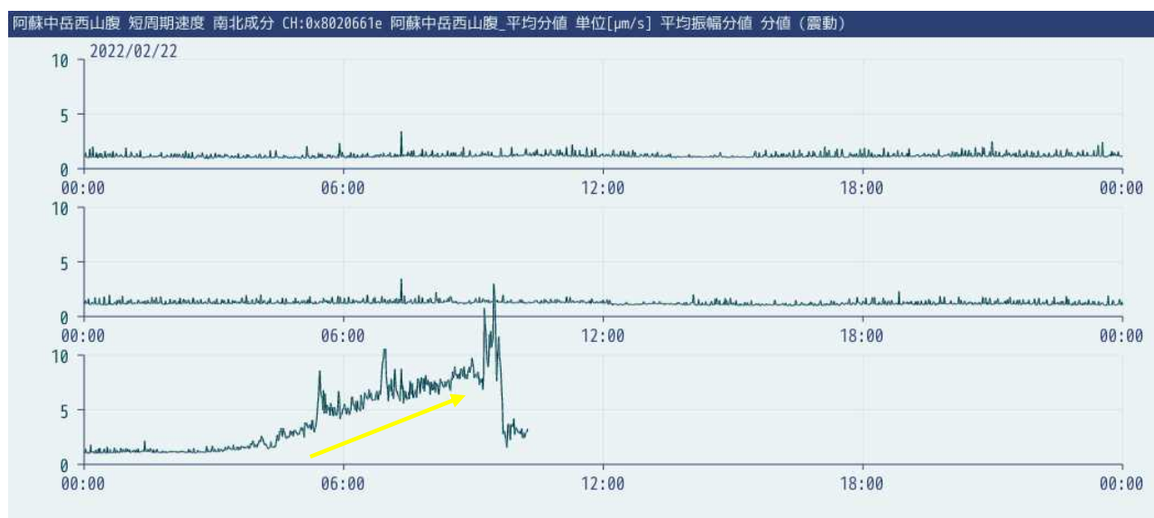
図2 阿蘇山 中岳西山腹での1分間平均振幅
