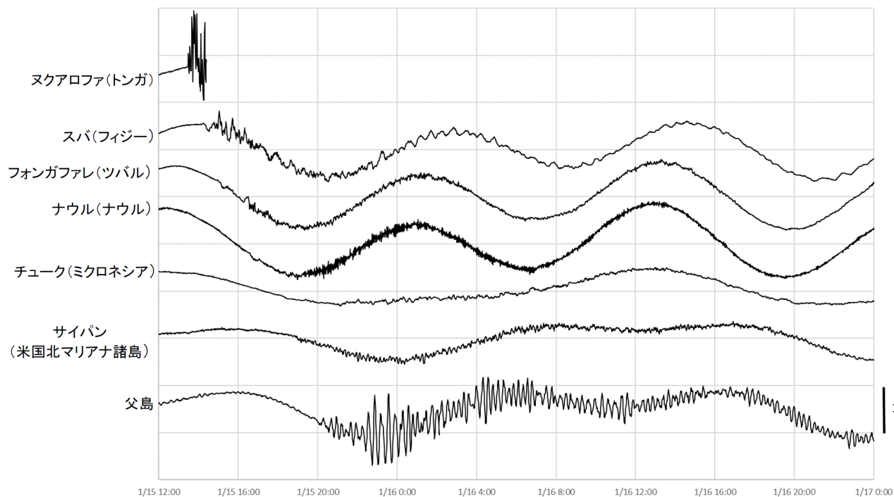
図 3-6 主な海外観測点の潮位波形（トンガー日本間の経路上の観測点） （2022 年 1 月 15 日 12 時～1 月 17 日 00 時（日本時間））
