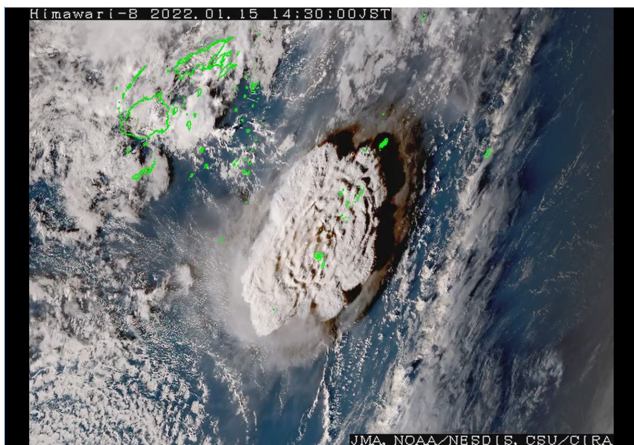
図４－１ 気象衛星ひまわりによって撮影された1月15日の噴火に伴う噴煙（2022年1月15日14時30分（日本時間）、現地時刻18時30分）
