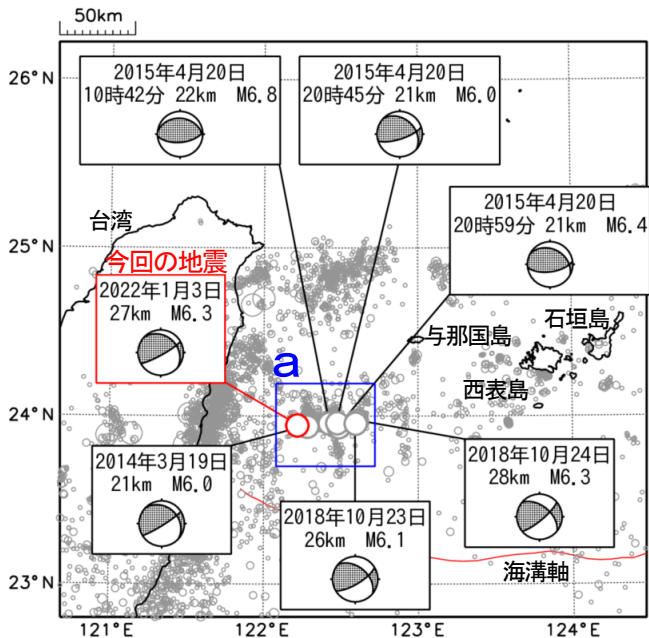
震央分布図 (2009年9月1日～2022年1月3日、 深さ0～50km、 M \geq 3.0 ) 2022年1月の地震を赤く表示 図中の発震機構はCMT解
