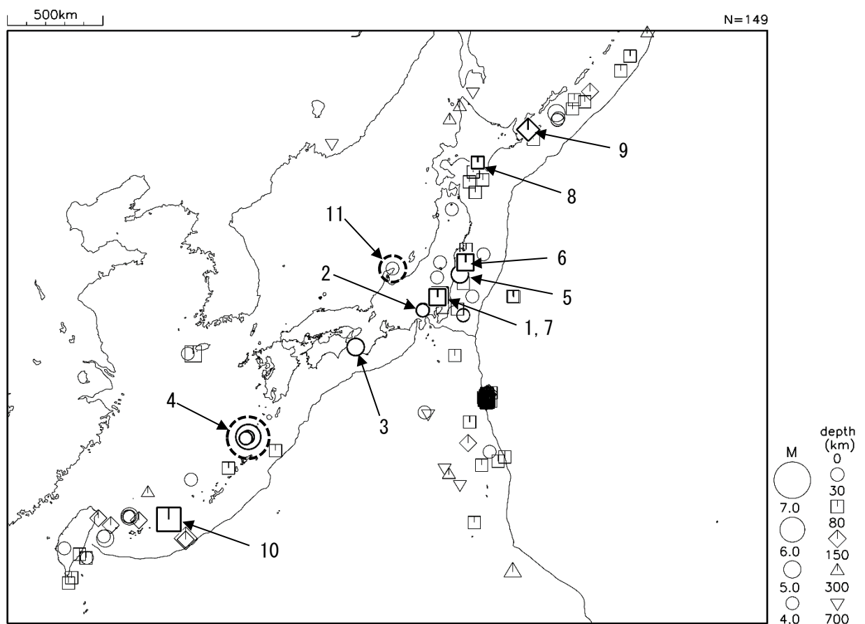
令和3年12月に発生したM4.0以上の地震（図中の番号は、表の番号に対応）
