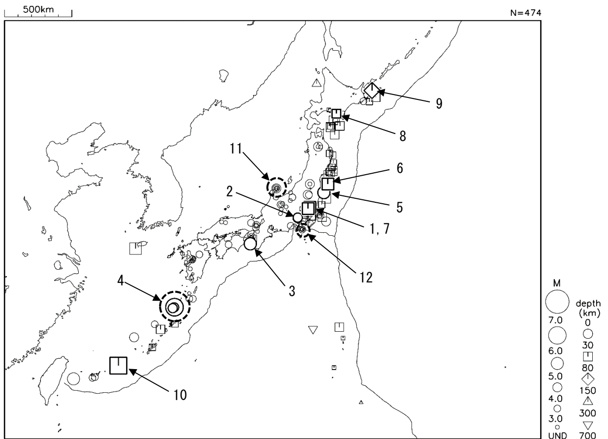
令和3年12月に震度1以上を観測した地震（図中の番号は、表の番号に対応）
