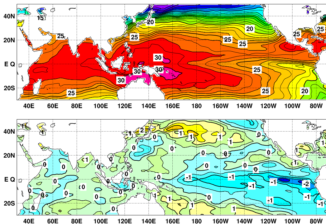
図4 2021年12月の海面水温図（上）及び平年偏差図（下）
