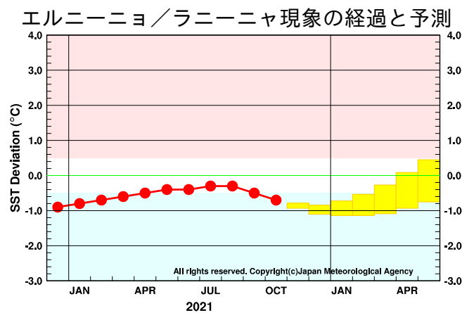
図 1 エルニーニョ監視海域の海面水温の基準値との差の 5 か月移動平均値 10 月までの経過（観測値）を折れ線グラフで、エルニーニョ予測モデルによる予測結果（70%の確率で入ると予想される範囲）をボックスで示している。指数が赤／青の範囲に入っている期間がエルニーニョ／ラニーニャ現象の発生期間である。エルニーニョ監視海域の海面水温の基準値はその年の前年までの 30 年間の各月の平均値。
