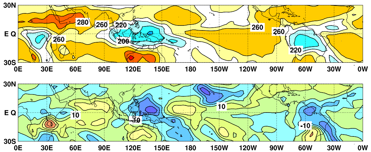
図 9 外向き長波放射量 (OLR) (上) 及び年偏差 (下) の分布図 (2021 年 12 月)
