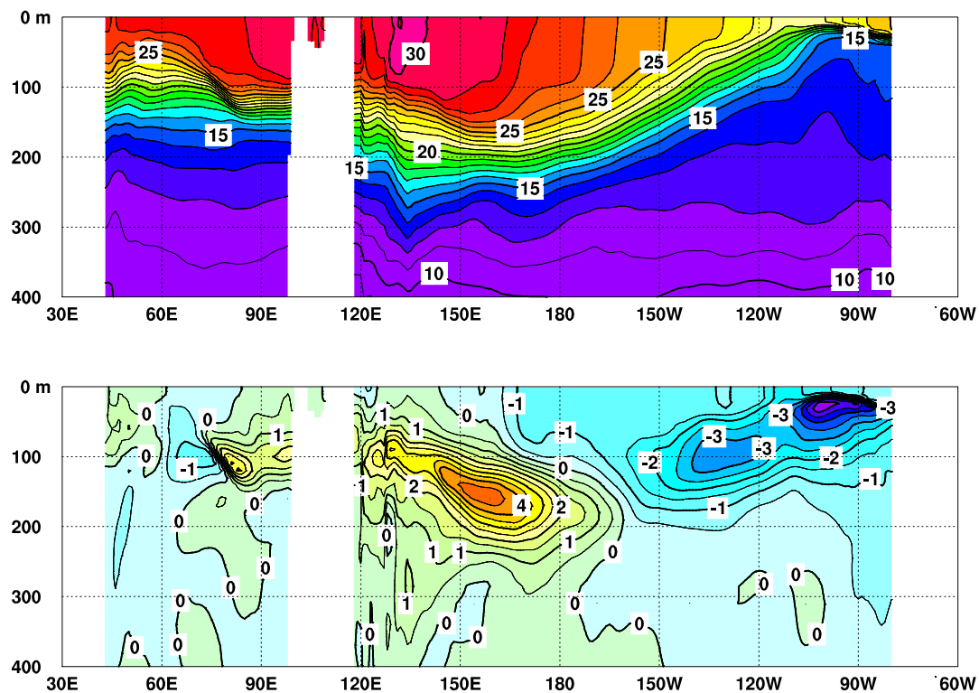
図5 2021年12月のインド洋から太平洋の赤道に沿った水温（上）及び平年偏差（下）の断面図
