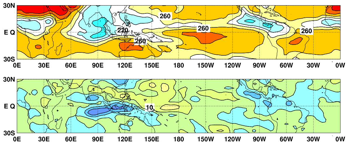
図 9 外向き長波放射量 (OLR) (上) 及び年偏差 (下) の分布図 (2021 年 8 月)
