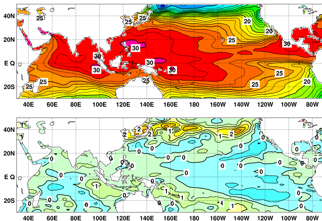
図4 2021年7月の海面水温図(上)及び平年偏差図(下)
