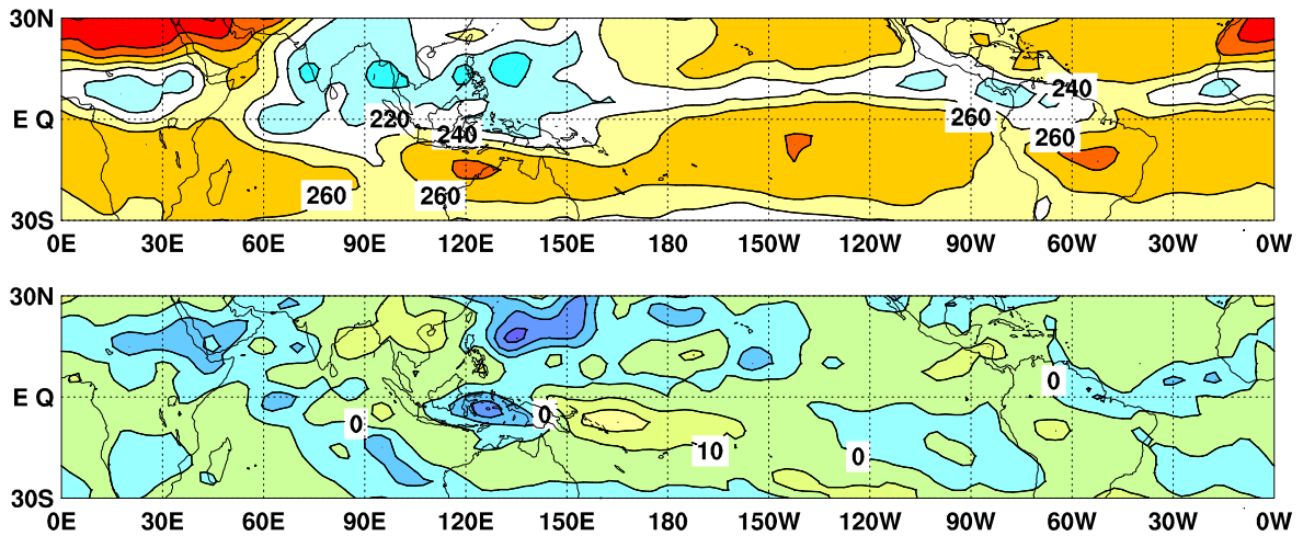
図9 外向き長波放射量 (OLR) (上) 及び年偏差 (下) の分布図 (2021年7月)
