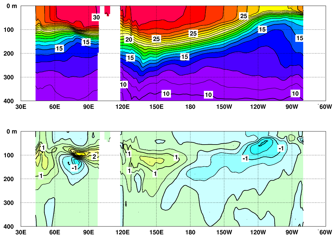
図5 2021年7月のインド洋から太平洋の赤道に沿った水温(上)及び平年偏差(下)の断面図
