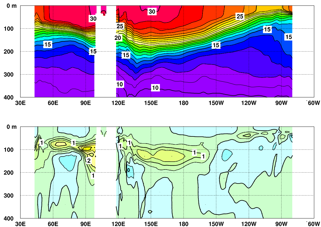
図5 2021年6月のインド洋から太平洋の赤道に沿った水温（上）及び平年偏差（下）の断面図
