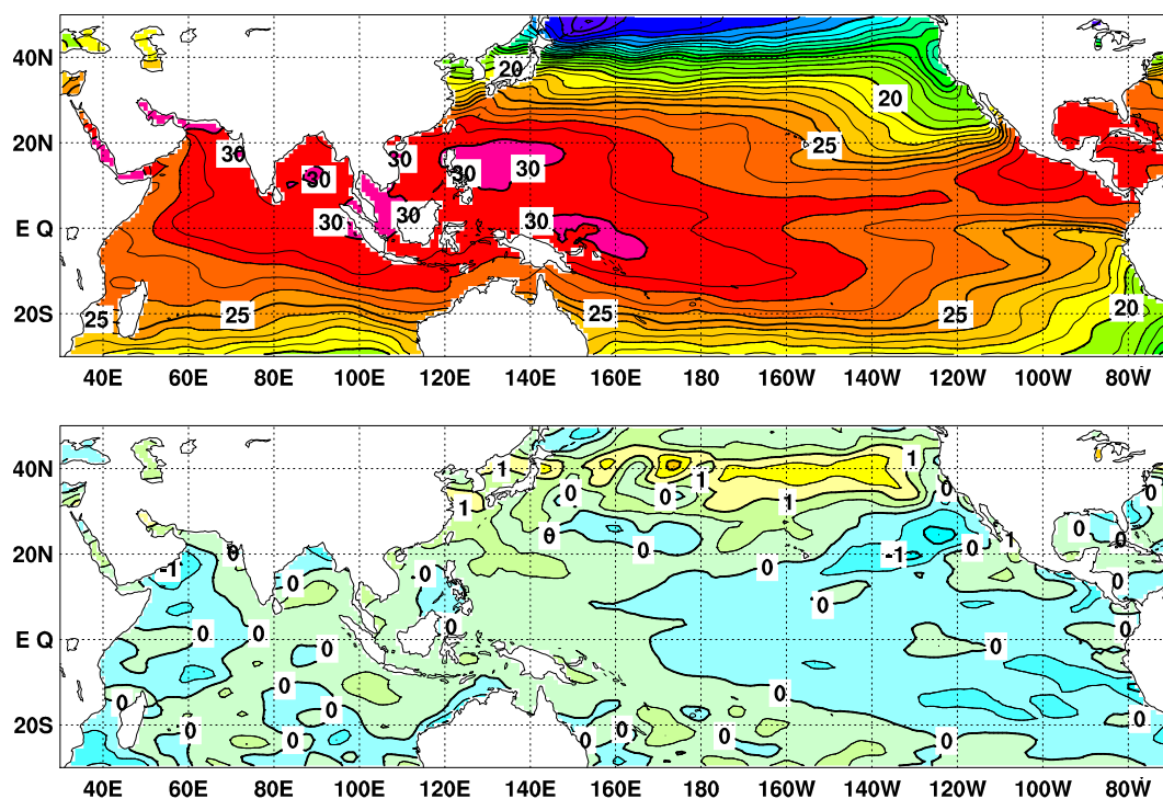
図4 2021年6月の海面水温図（上）及び平年偏差図（下）
