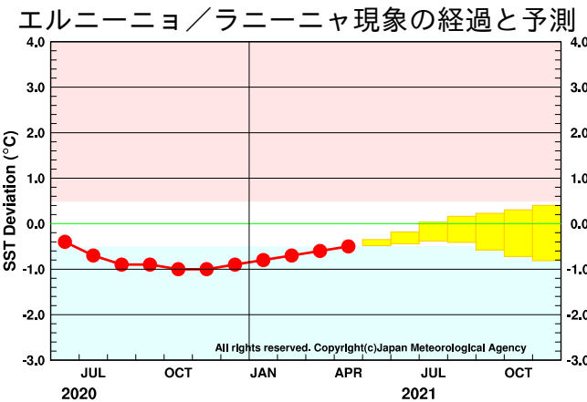
図 1 エルニーニョ監視海域の海面水温の基準値との差の 5 か月移動平均値 4 月までの経過（観測値）を折れ線グラフで、エルニーニョ予測モデルによる予測結果（70%の確率で入ると予想される範囲）をボックスで示している。指数が赤／青の範囲に入っている期間がエルニーニョ／ラニーニャ現象の発生期間である。エルニーニョ監視海域の海面水温の基準値はその年の前年までの 30 年間の各月の平均値。
