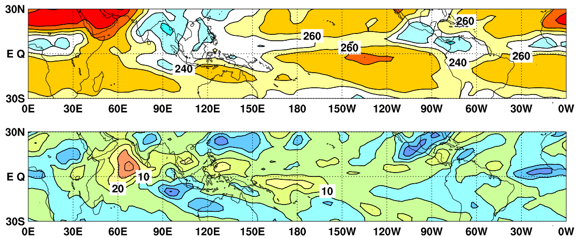
図 9 外向き長波放射量 (OLR) (上) 及び年間偏差 (下) の分布図 (2021 年 6 月)
