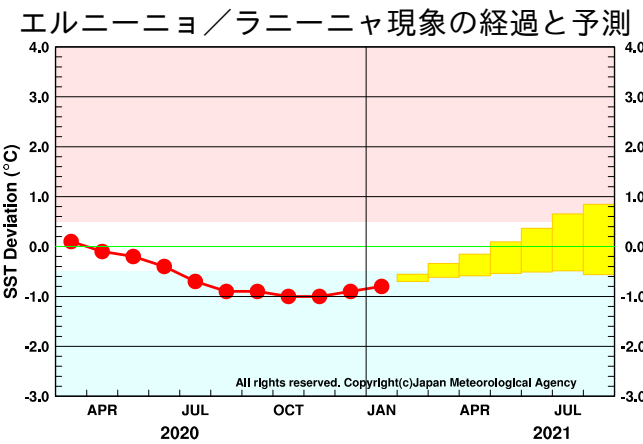
図 1 エルニーニョ監視海域の海面水温の基準値との差の 5 か月移動平均値 1 月までの経過（観測値）を折れ線グラフで、エルニーニョ予測モデルによる予測結果（70%の確率で入ると予想される範囲）をボックスで示している。指数が赤／青の範囲に入っている期間がエルニーニョ／ラニーニャ現象の発生期間である。エルニーニョ監視海域の海面水温の基準値はその年の前年までの 30 年間の各月の平均値。
