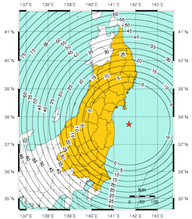
警報第 2 報発表から主要動到達までの 時間及び警報発表対象地域の分布図
