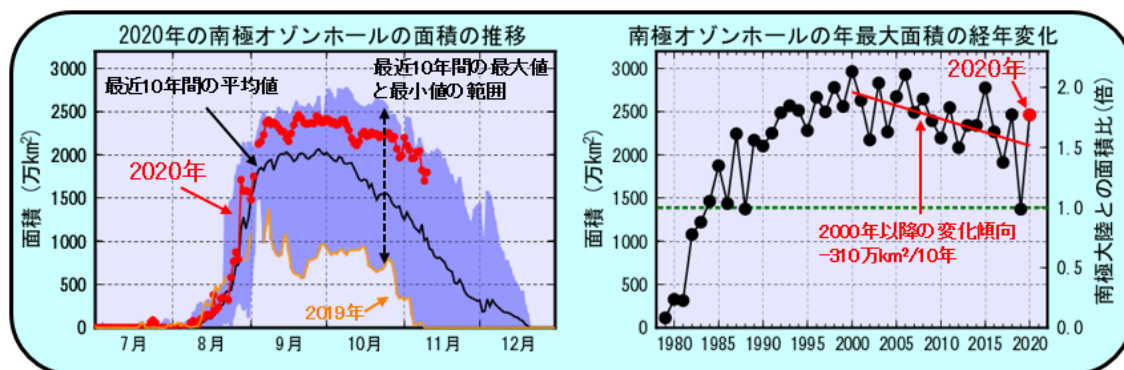
図 南極オゾンホールの2020年の面積の推移と年最大面積の経年変化
