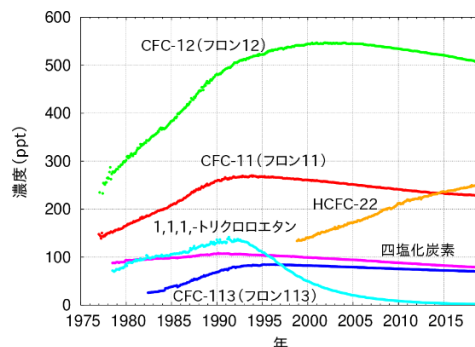
参考図 主なオゾン層破壊物質の月平均濃度の経年変化（世界の観測所の平均） 世界気象機関温室効果ガス世界資料センター（気象庁が運営）のデータにより作成。
