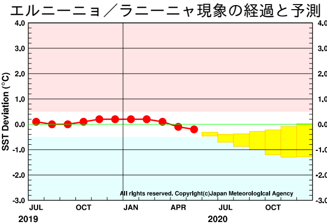
図 1 エルニーニョ監視海域の海面水温の基準値との差の 5 か月移動平均値 5 月までの経過（観測値）を折れ線グラフで、エルニーニョ予測モデルによる予測結果（70%の確率で入ると予想される範囲）をボックスで示している。指数が赤／青の範囲に入っている期間がエルニーニョ／ラニーニャ現象の発生期間である。エルニーニョ監視海域の海面水温の基準値はその年の前年までの 30 年間の各月の平均値。
