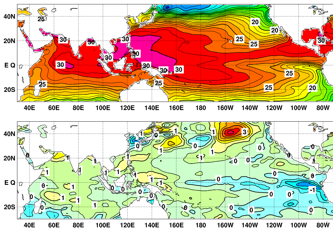
図4 2020年7月の海面水温図（上）及び平年偏差図（下）
