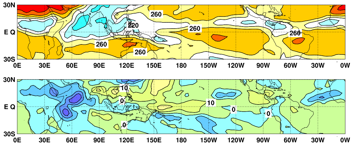
図 9 外向き長波放射量 (OLR) (上) 及び年偏差 (下) の分布図 (2020 年 7 月)
