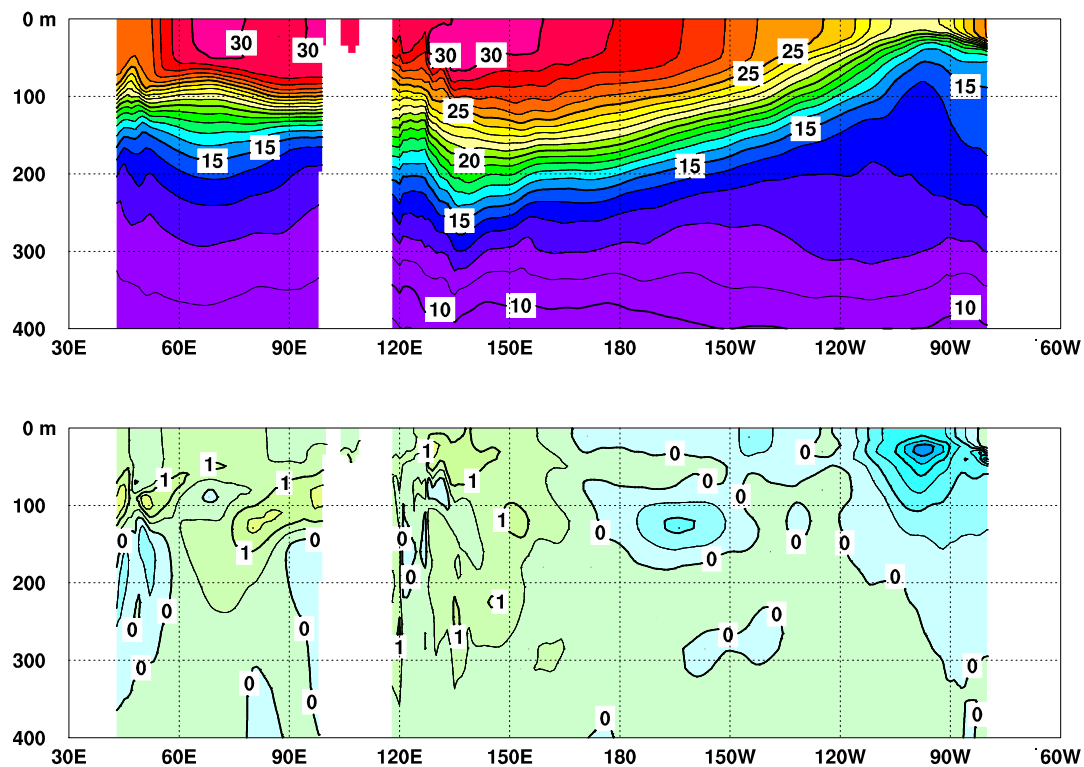
図5 2020年7月のインド洋から太平洋の赤道に沿った水温（上）及び平年偏差（下）の断面図
