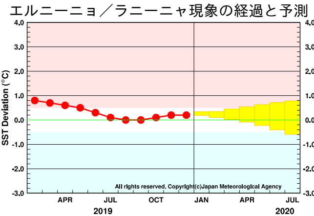
図 1 エルニーニョ監視海域の海面水温の基準値との差の 5 か月移動平均値 12 月までの経過（観測値）を折れ線グラフで、エルニーニョ予測モデルによる予測結果（70%の確率で入ると予想される範囲）をボックスで示している。指数が赤／青の範囲に入っている期間がエルニーニョ／ラニーニャ現象の発生期間である。エルニーニョ監視海域の海面水温の基準値はその年の前年までの 30 年間の各月の平均値。
