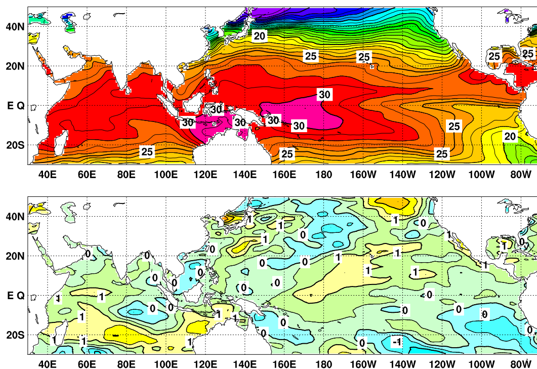
図4 2019年12月の海面水温図（上）及び平年偏差図（下）
