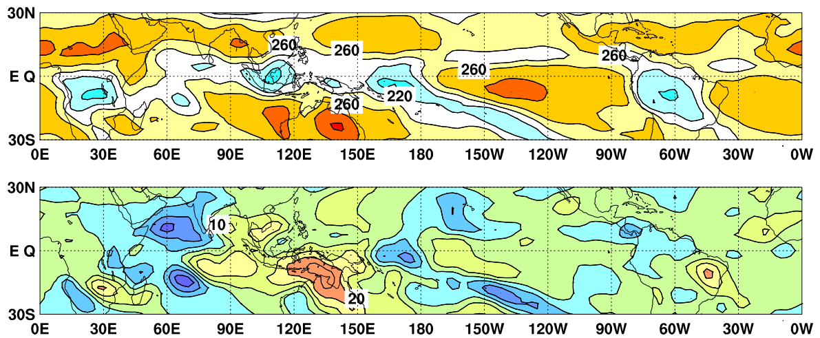
図 9 外向き長波放射量 (OLR) (上) 及び平年偏差 (下) の分布図 (2019 年 12 月)
