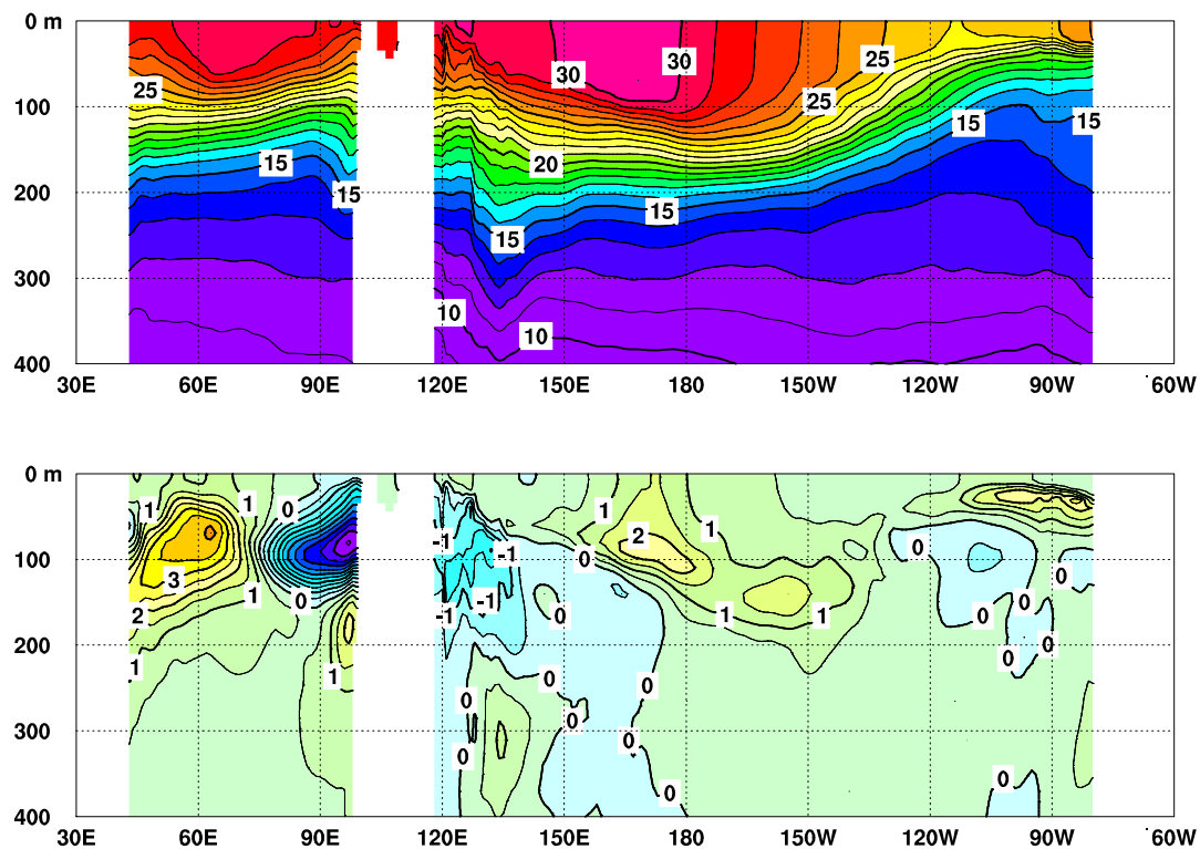
図5 2019年12月のインド洋から太平洋の赤道に沿った水温（上）及び平年偏差（下）の断面図
