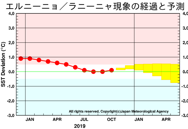
図 1 エルニーニョ監視海域の海面水温の基準値との差の 5 か月移動平均値 10 月までの経過（観測値）を折れ線グラフで、エルニーニョ予測モデルによる予測結果（70%の確率で入ると予想される範囲）をボックスで示している。指数が赤／青の範囲に入っている期間がエルニーニョ／ラニーニャ現象の発生期間である。エルニーニョ監視海域の海面水温の基準値はその年の前年までの 30 年間の各月の平均値。
