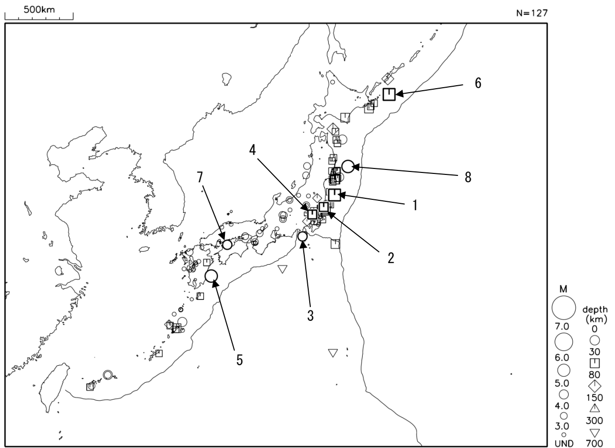
令和元年 11 月に震度 1 以上を観測した地震（図中の番号は、表の番号に対応）
