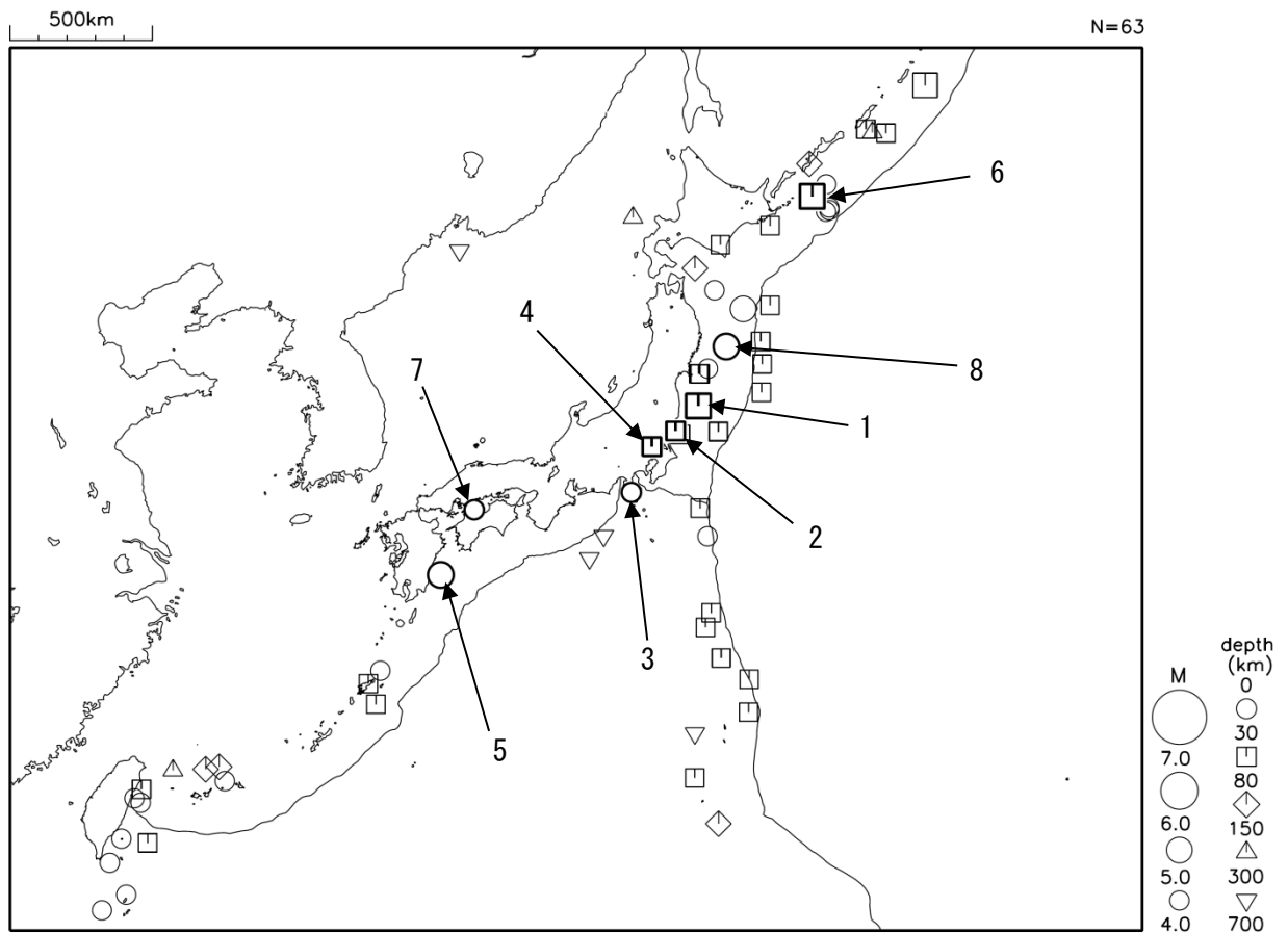
令和元年 11 月に発生した M4.0 以上の地震（図中の番号は、表の番号に対応）
