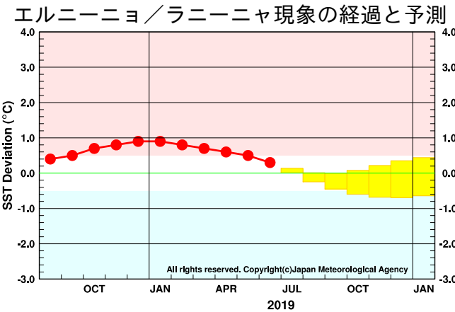
図 1 エルニーニョ監視海域の海面水温の基準値との差の 5 か月移動平均値 6 月までの経過（観測値）を折れ線グラフで、エルニーニョ予測モデルによる予測結果（70%の確率で入ると予想される範囲）をボックスで示している。指数が赤／青の範囲に入っている期間がエルニーニョ／ラニーニャ現象の発生期間である。エルニーニョ監視海域の海面水温の基準値はその年の前年までの 30 年間の各月の平均値。
