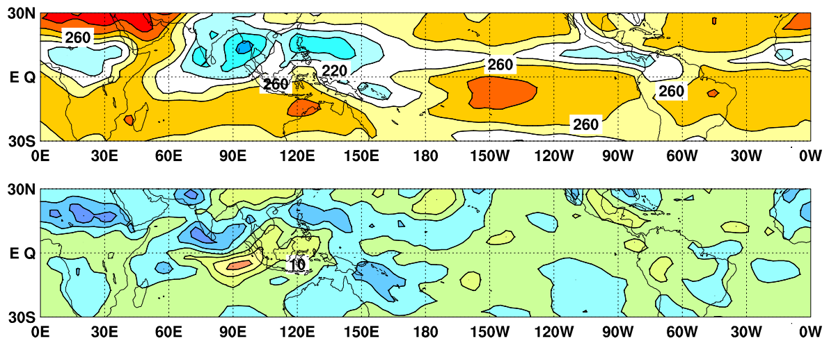
図 9 外向き長波放射量 (OLR) (上) 及び年偏差 (下) の分布図 (2019 年 8 月)
