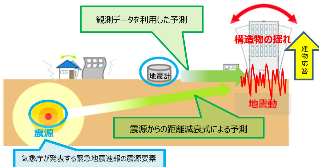
図 8 震源あるいは観測データから予測ポイントの長周期地震動や構造物の揺れを予測する過程のイメージ
