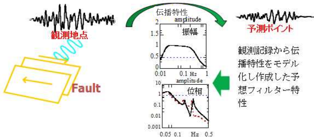
図 18 モデル化した伝播特性を使った地震動予測イメージ
