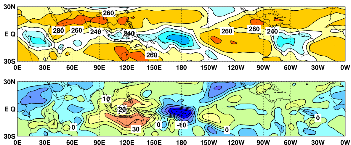
図 9 外向き長波放射量 (OLR) (上) 及び年偏差 (下) の分布図 (2019 年 2 月)
