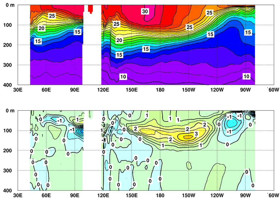
図5 2019年2月のインド洋から太平洋の赤道に沿った水温（上）及び平年偏差（下）の断面図
