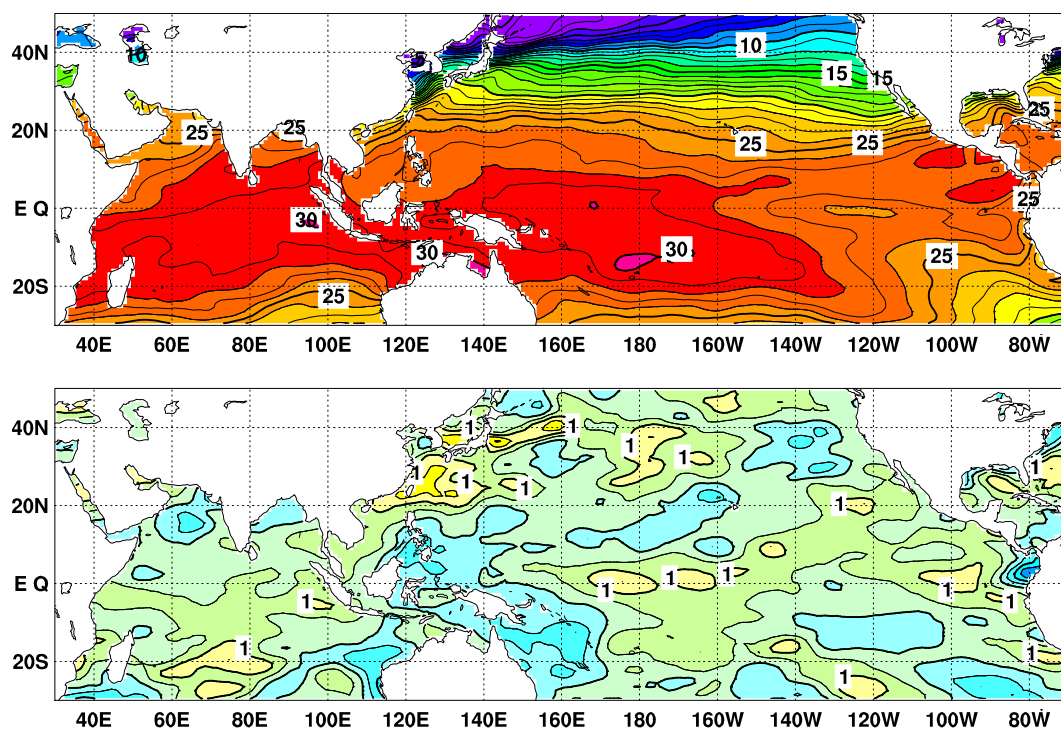
図4 2019年2月の海面水温図（上）及び平年偏差図（下）
