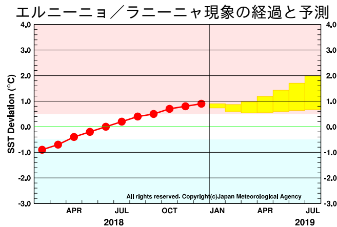
図 1 エルニーニョ監視海域の海面水温の基準値との差の 5 か月移動平均値 12 月までの経過（観測値）を折れ線グラフで、エルニーニョ予測モデルによる予測結果（70%の確率で入ると予想される範囲）をボックスで示している。指数が赤／青の範囲に入っている期間がエルニーニョ／ラニーニャ現象の発生期間である。エルニーニョ監視海域の海面水温の基準値はその年の前年までの 30 年間の各月の平均値。
