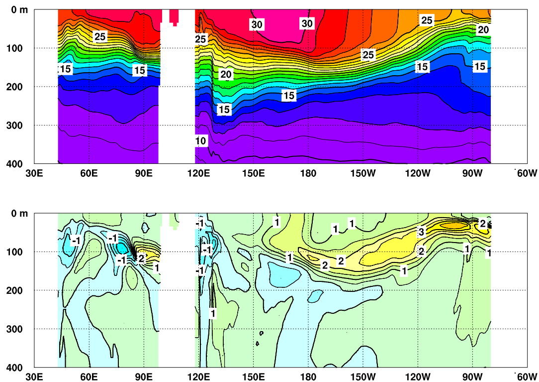
図5 2018年12月のインド洋から太平洋の赤道に沿った水温（上）及び平年偏差（下）の断面図
