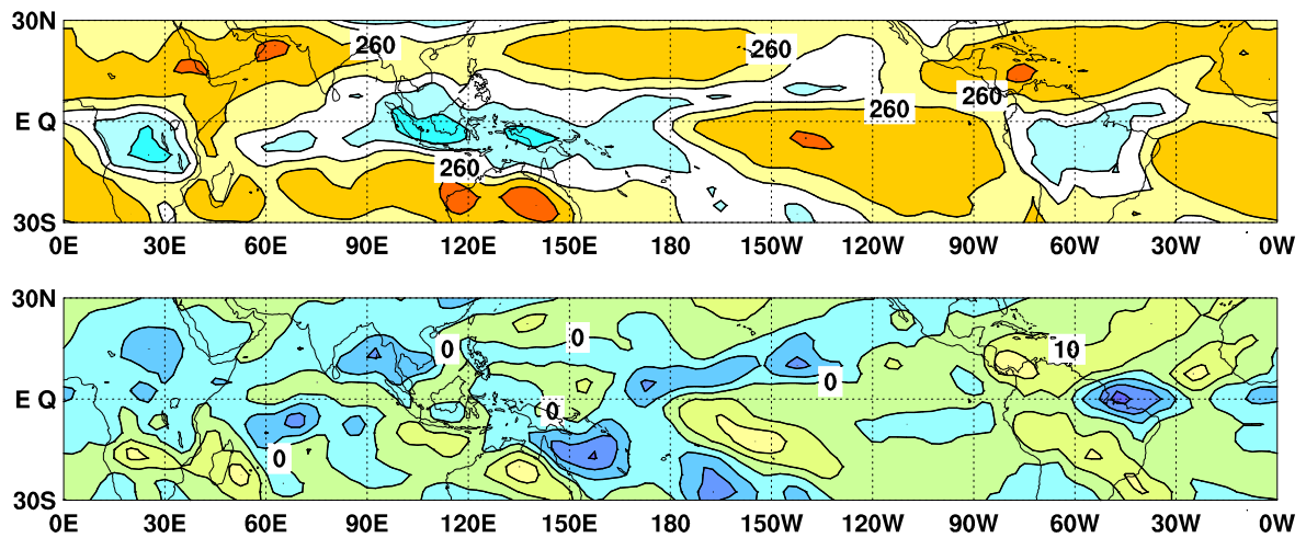
図 9 外向き長波放射量 (OLR) (上) 及び平年偏差 (下) の分布図 (2018 年 12 月)
