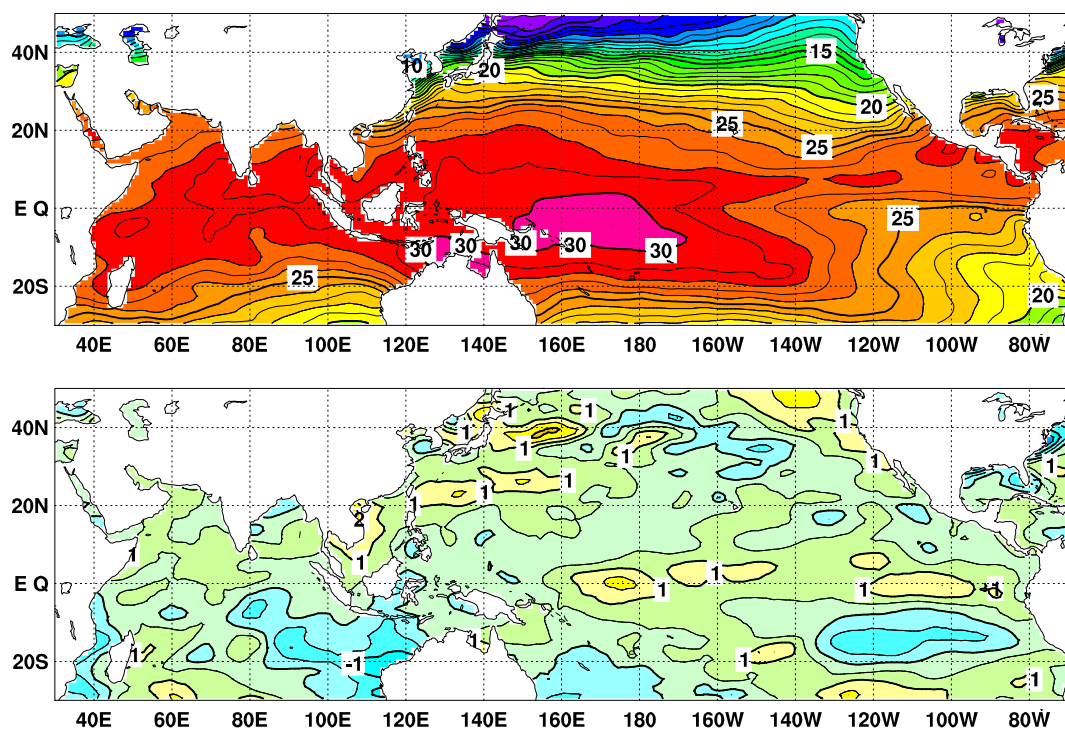
図4 2018年12月の海面水温図（上）及び平年偏差図（下）
