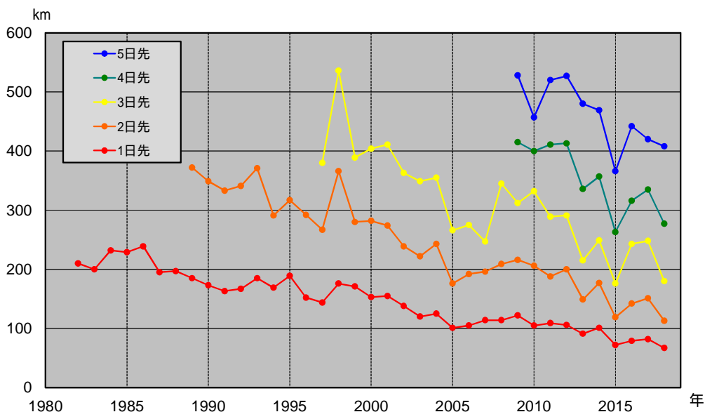
図4 台風進路予報誤差の経年変化(12月21日現在) 赤：1日先、橙：2日先、黄：3日先、緑：4日先、青：5日先 台風第27号～第29号は速報値
