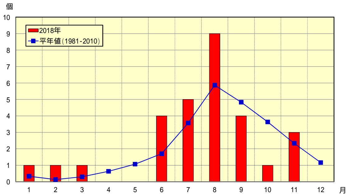
図2 2018年（平成30年）の月別発生数(12月21日現在) 赤：発生数、青：平年値（1981～2010年の30年平均値）
