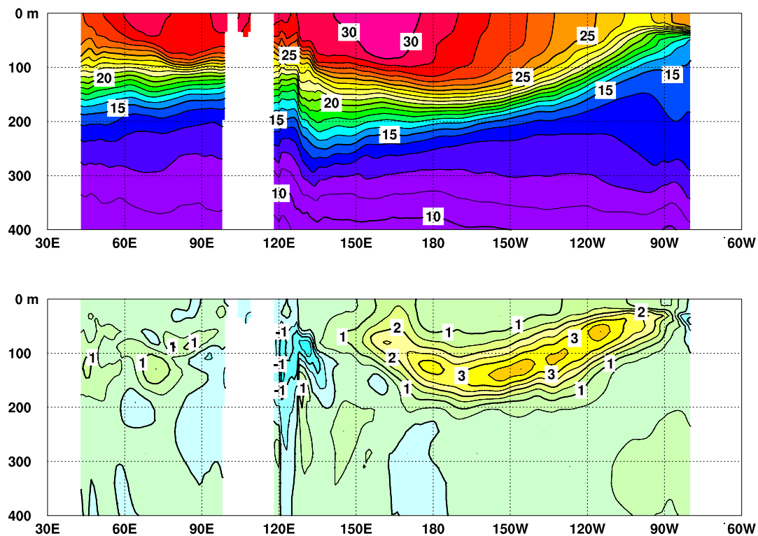
図5 2018年10月のインド洋から太平洋の赤道に沿った水温(上)及び平年偏差(下)の断面図
