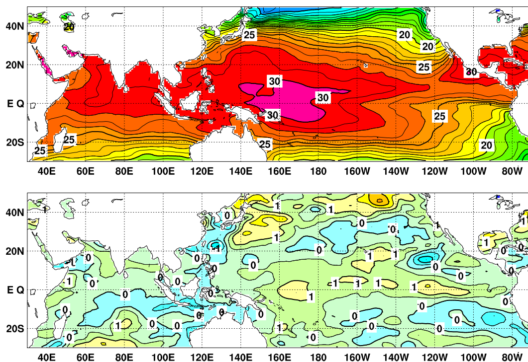
図4 2018年10月の海面水温図(上)及び平年偏差図(下)
