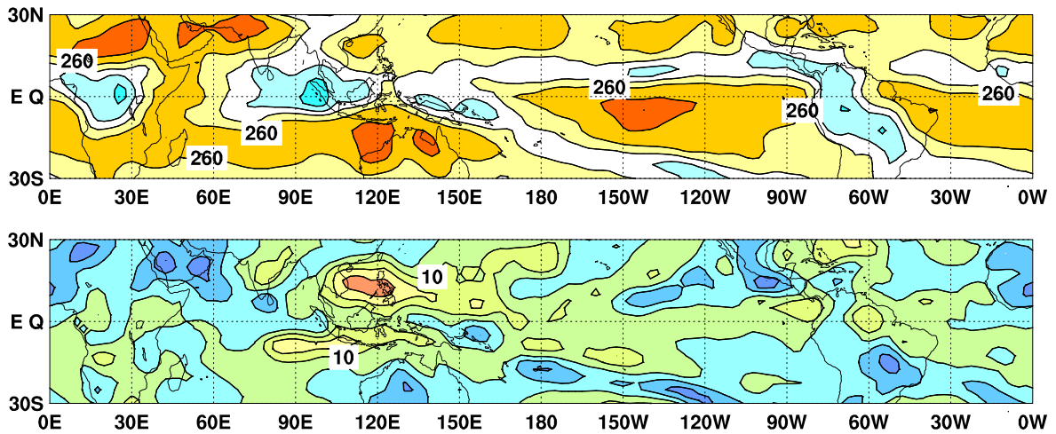
図9 外向き長波放射量 (OLR) (上) 及び平年偏差 (下) の分布図 (2018年10月)
