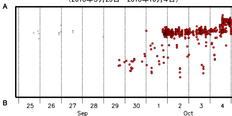
震央分布図の領域a内の時空間分布図(A-B投影) (2018年9月25日～2018年10月4日)
