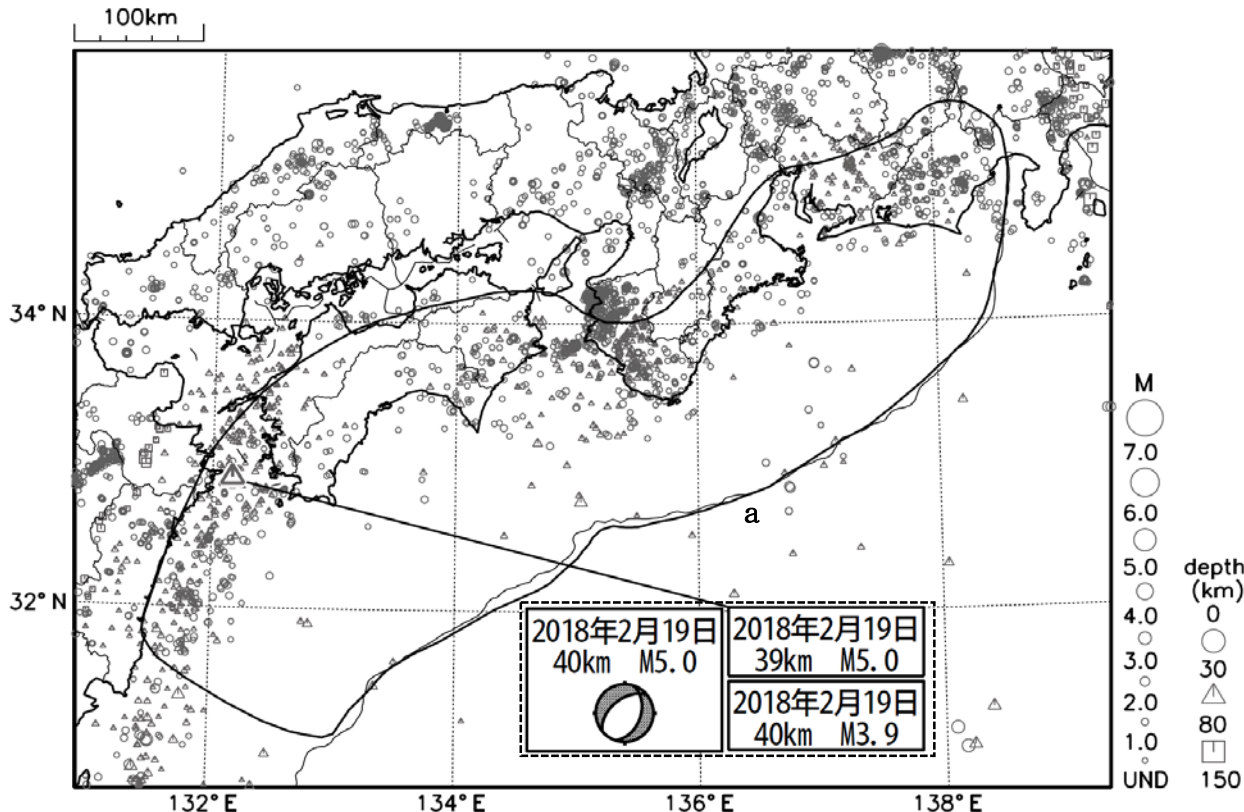
図1 震央分布図（2018年2月1日～2月28日、深さ0～150km、Mすべて、図中の領域aは、南海トラフ巨大地震の想定震源域） ※図中の吹き出しは、領域a内のM3.5以上、それ以外の陸域M5.0以上・海域M6.0以上とその他の主な地震
