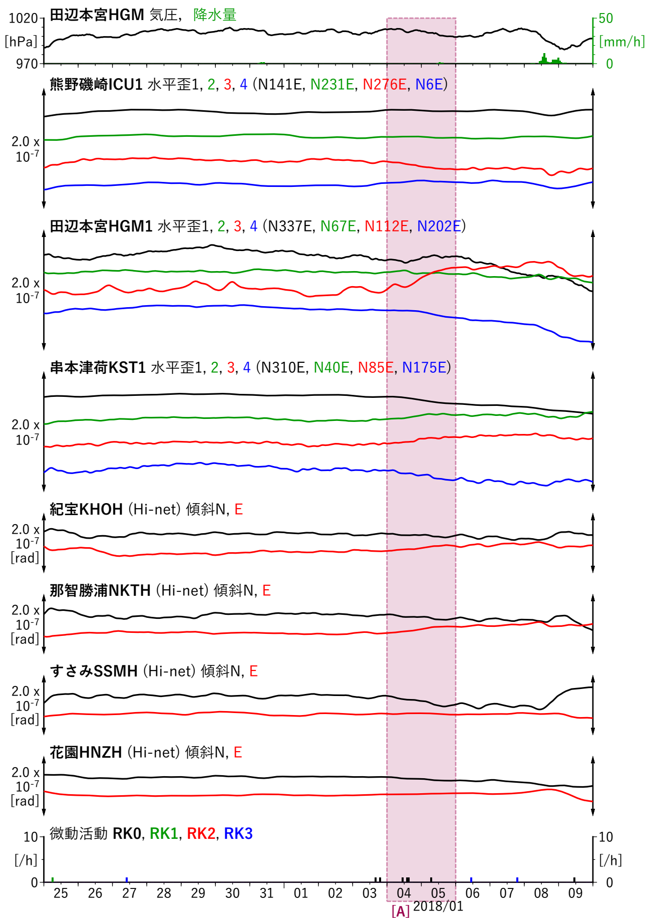
図2 歪・傾斜の時間変化 (2017/12/25 00:00 - 2018/01/10 00:00 (JST))
