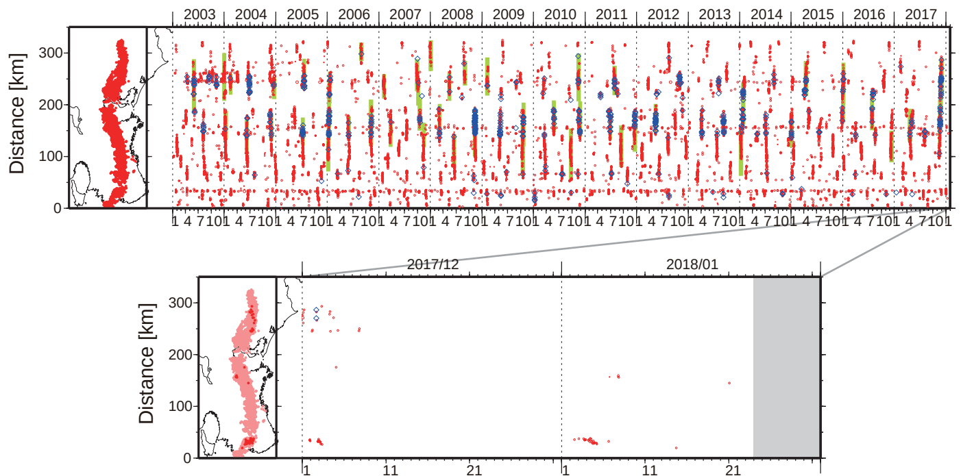
図 1. 紀伊半島・東海地域における 2003 年 1 月～2018 年 1 月 23 日までの深部低周波微動の時空間分布 (上図). 赤丸はエンベロップ相関・振幅ハイブリッド法 (Maeda and Obara, 2009) およびクラスタ処理 (Obara et al., 2010) によって 1 時間毎に自動処理された微動分布の重心である. 青菱形は周期 20 秒に卓越する超低周波地震 (Ito et al., 2007) である. 黄緑色の太線はこれまでに検出された短期的スロースリップイベント (SSE) を示す. 下図は 2017 年 12 月～2018 年 1 月の拡大図である. 12 月下旬以降の顕著な活動としては、1 月 2～6 日頃に和歌山県中部でやや活発な活動が発生し、やや西方向への活動域の移動がみられた. また、1 月 6～7 日頃には三重県北部において、ごく小規模な活動がみられた. 1 月 23 日 18:31 頃 (日本標準時) にアラスカ湾付近で発生した Mw7.9(USGS) の地震後の 19:05～19:20 頃に、ハイブリッド法により微動活動が愛知県中部で検出されている (図 3).
