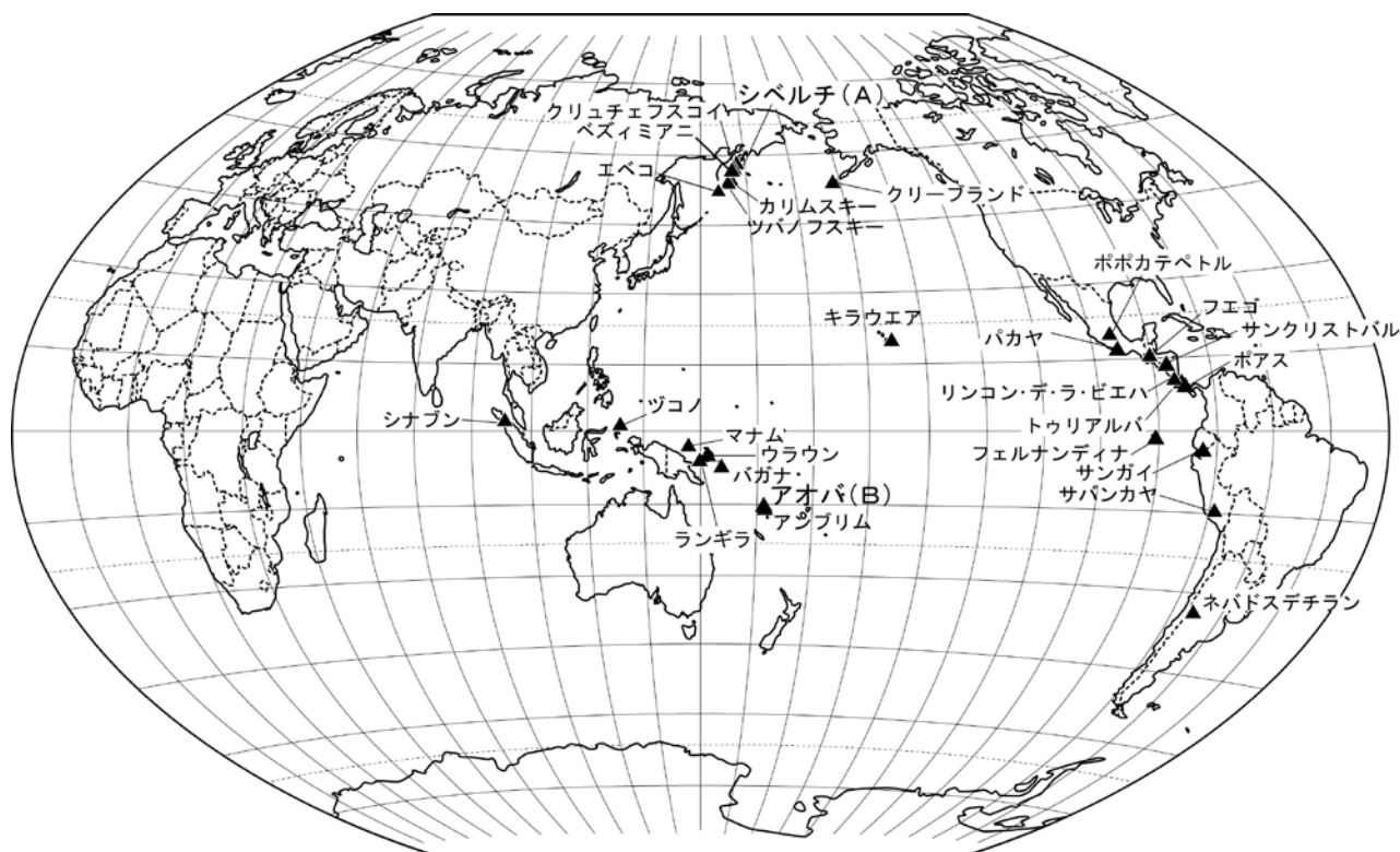
図 平成 29 年（2017 年）9 月に噴火した主な火山（日本を除く）*
