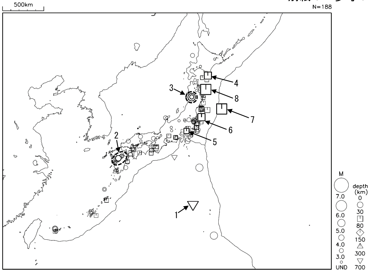
図 1 平成 29 年 9 月に震度 1 以上を観測した地震 (図中の番号は、「平成 29 年 9 月の主な地震活動」の表の番号に対応する主な地震)
