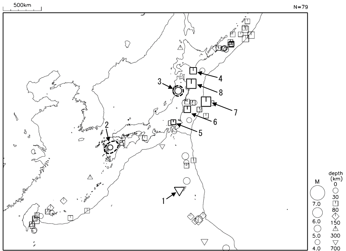
図 2 平成 29 年 9 月に発生した M4.0 以上の地震 (図中の番号は、「平成 29 年 9 月の主な地震活動」の表の番号に対応する主な地震)
