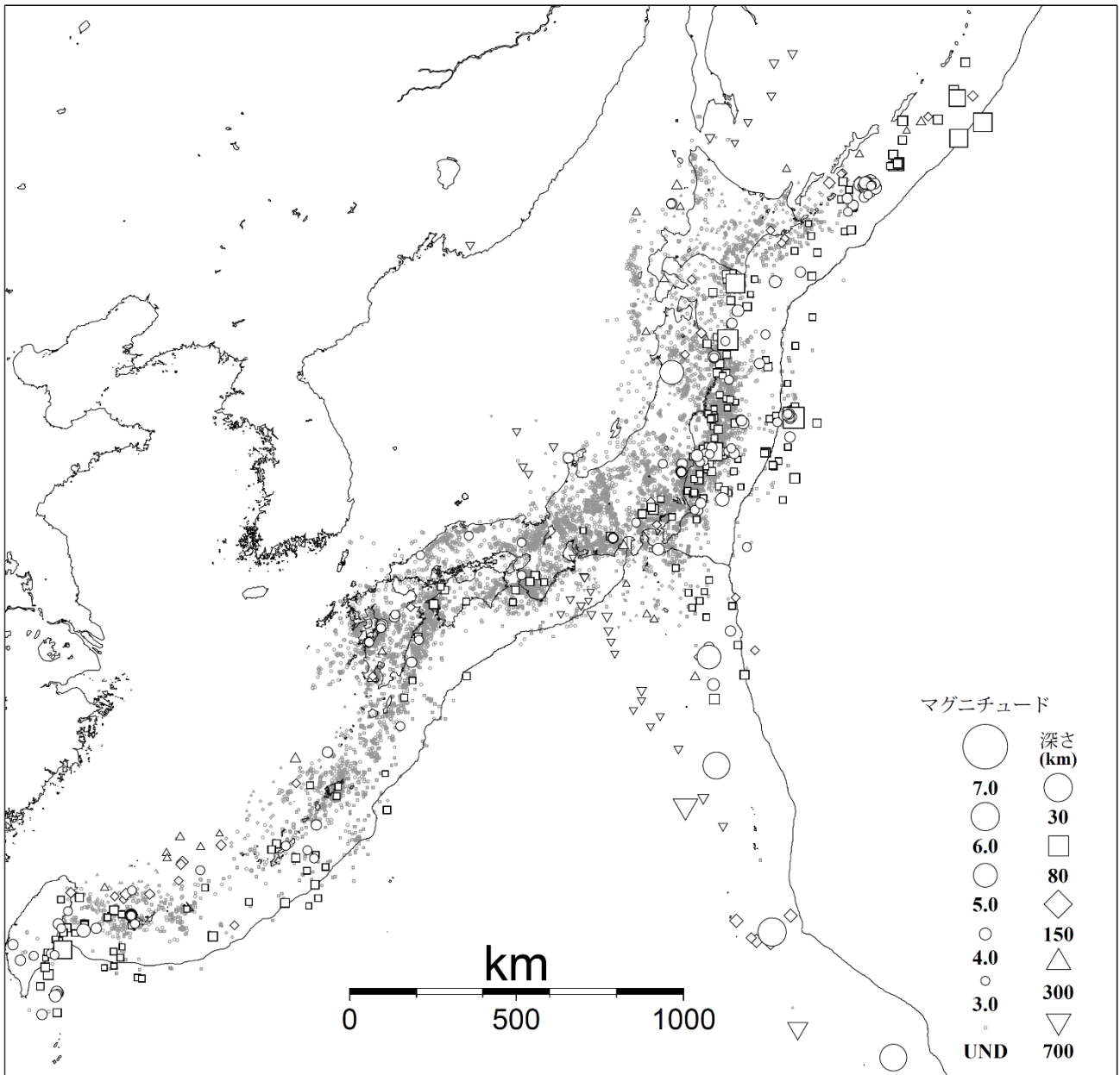
図3 気象庁が震源を決定した日本付近の平成 29 年 9 月の地震の震央分布 (M3.0 以上の地震については白抜きで示す)
