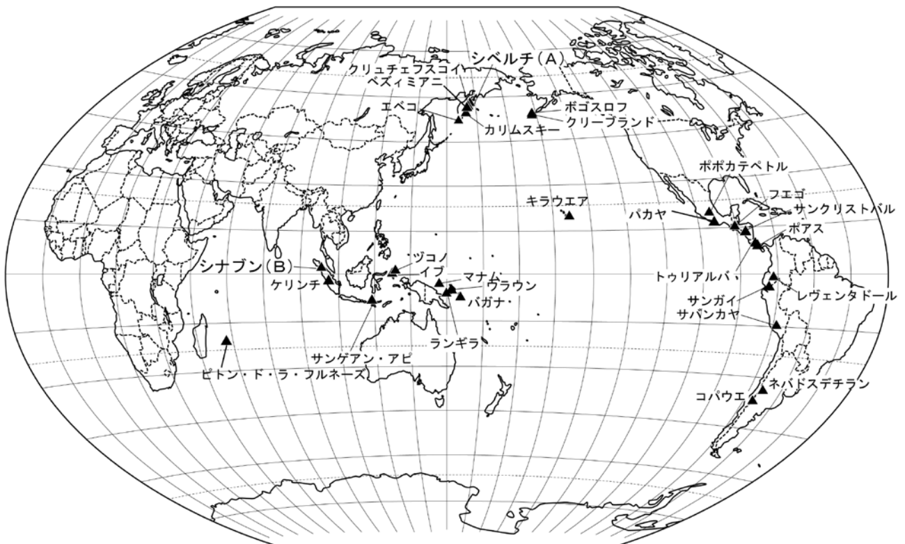
図 平成 29 年（2017 年）8 月に噴火した主な火山（日本を除く）*
