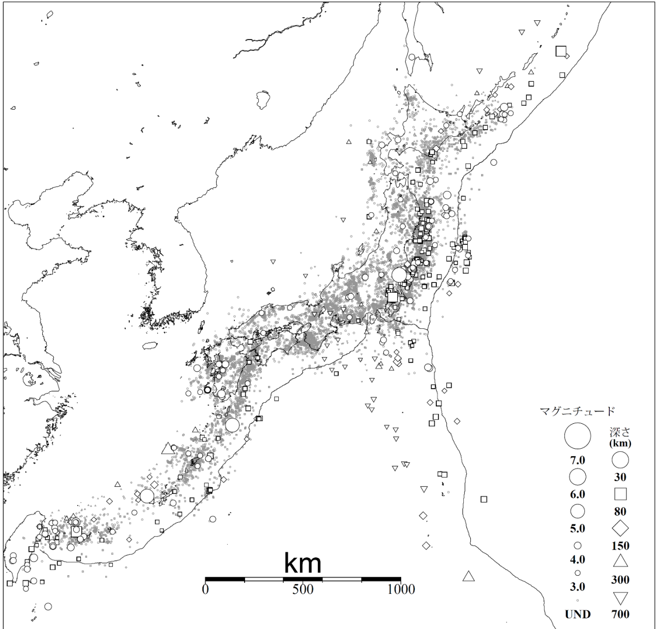
図3 気象庁が震源を決定した日本付近の平成29年8月の地震の震央分布 (M3.0以上の地震については白抜きで示す)
