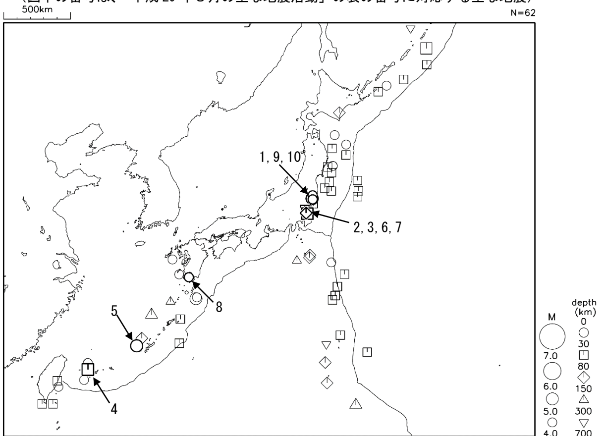
図2 平成29年8月に発生したM4.0以上の地震 (図中の番号は、「平成29年8月の主な地震活動」の表の番号に対応する主な地震)
