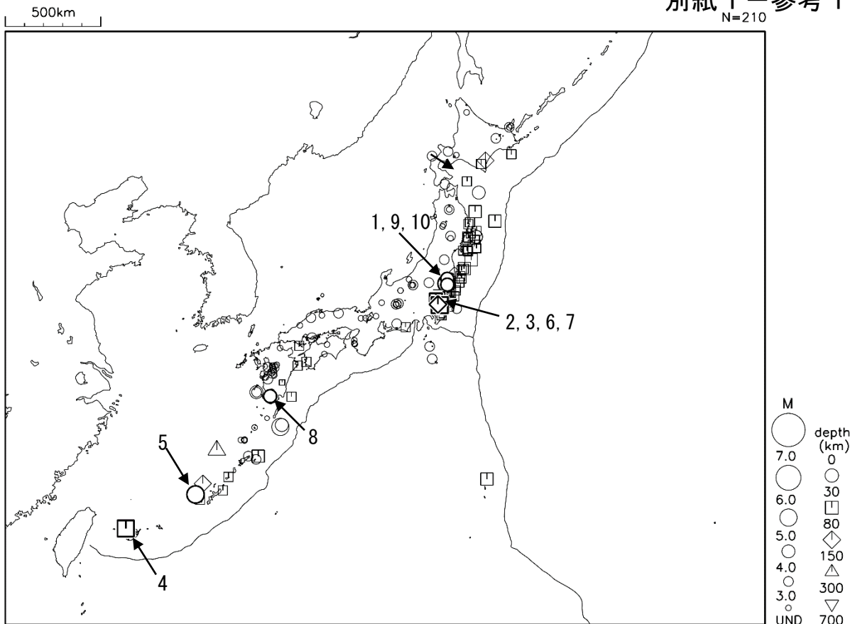
図1 平成29年8月に震度1以上を観測した地震 (図中の番号は、「平成29年8月の主な地震活動」の表の番号に対応する主な地震)
