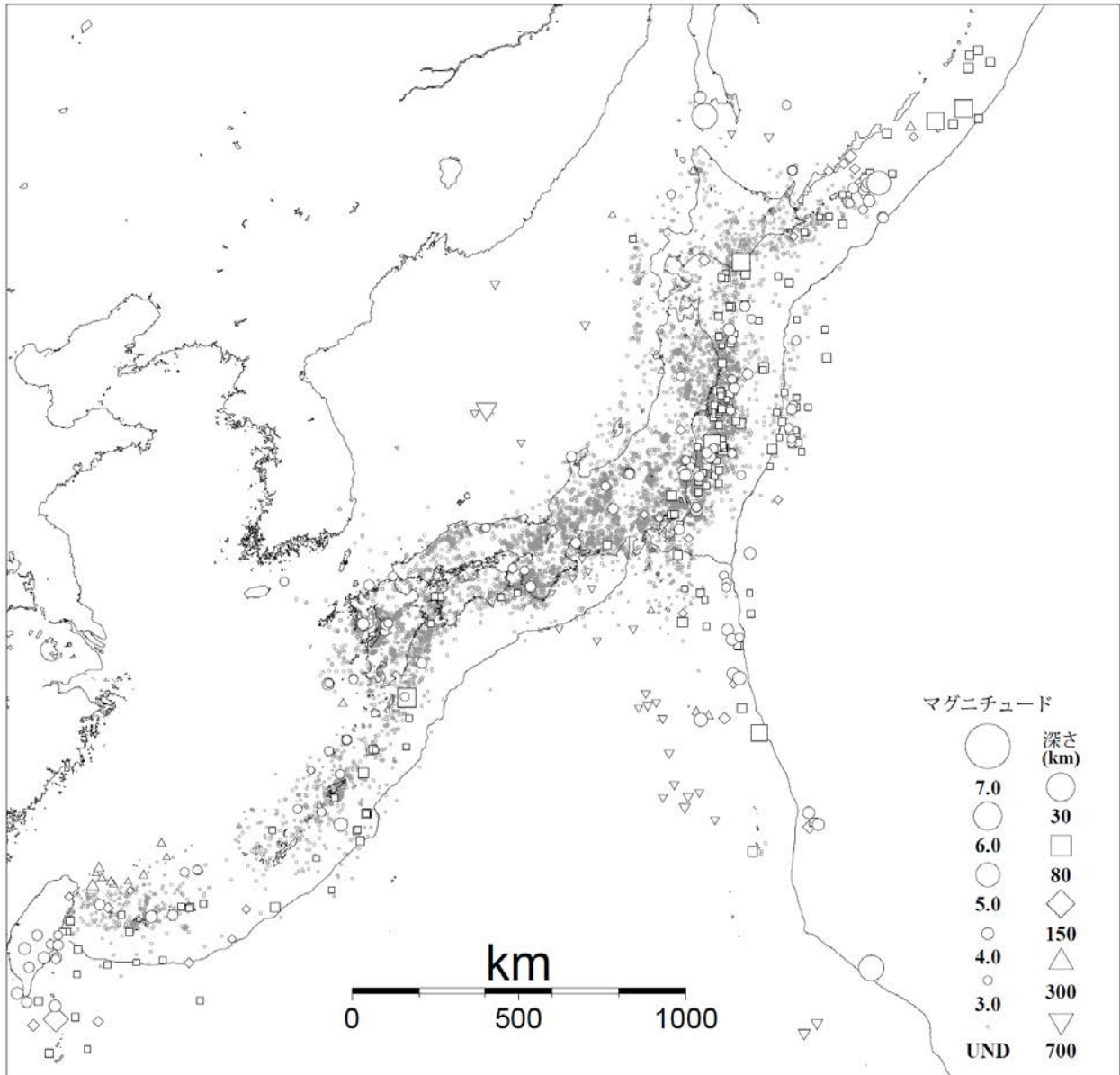
図3 気象庁が震源を決定した日本付近の平成 29 年 4 月の地震の震央分布 (M3.0 以上の地震については白抜きで示す)
