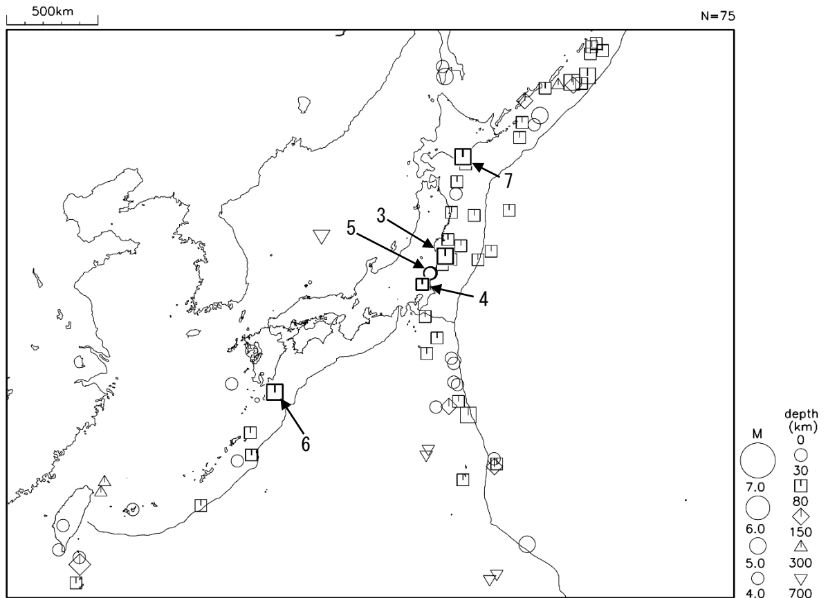
図 2 平成 29 年 4 月に発生した M4.0 以上の地震 (図中の番号は、「平成 29 年 4 月の主な地震活動」の表の番号に対応する主な地震)
