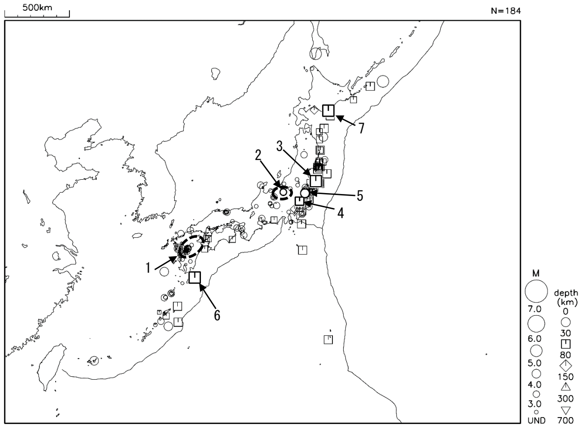
図 1 平成 29 年 4 月に震度 1 以上を観測した地震 (図中の番号は、「平成 29 年 4 月の主な地震活動」の表の番号に対応する主な地震)
