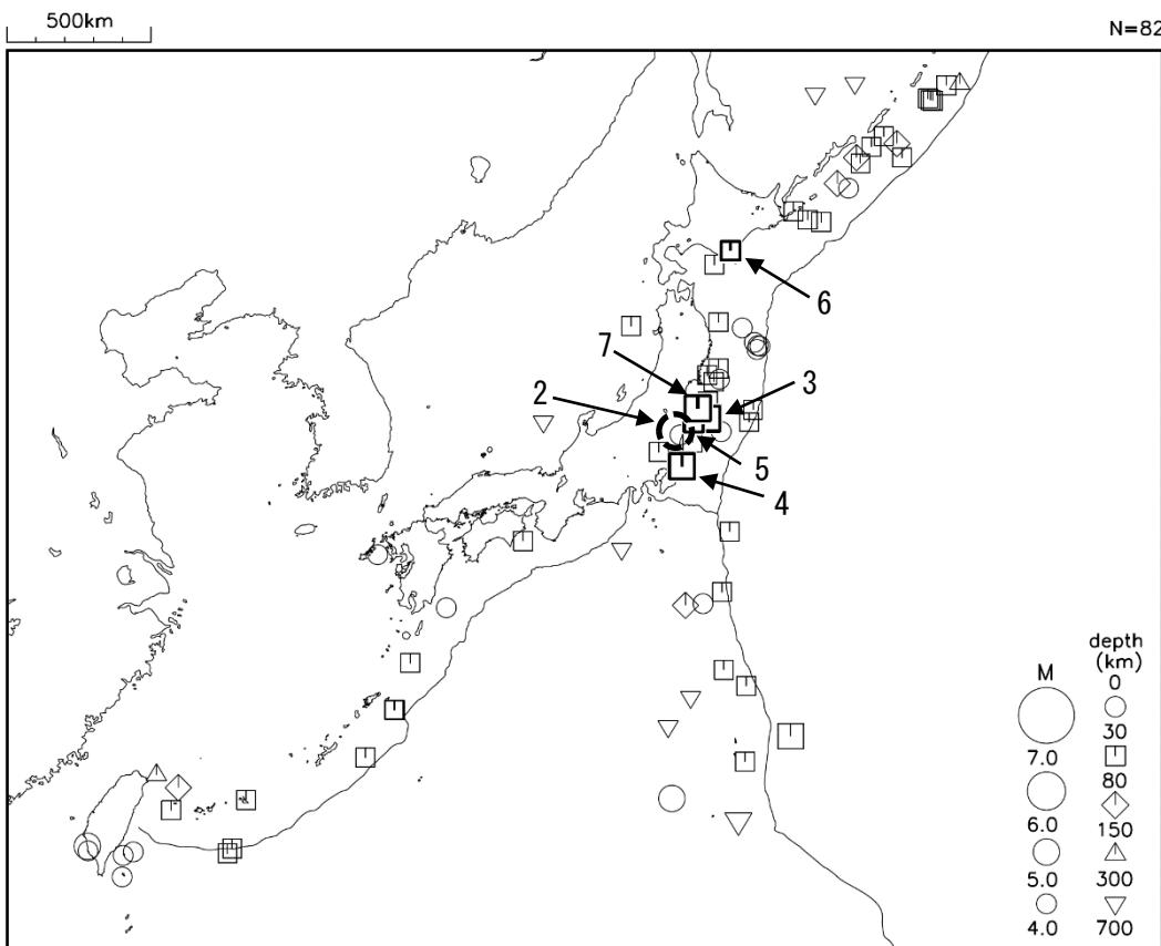
図 2 平成 29 年 2 月に発生した M4.0 以上の地震 (図中の番号は、「平成 29 年 2 月の主な地震活動」の表の番号に対応する主な地震)
