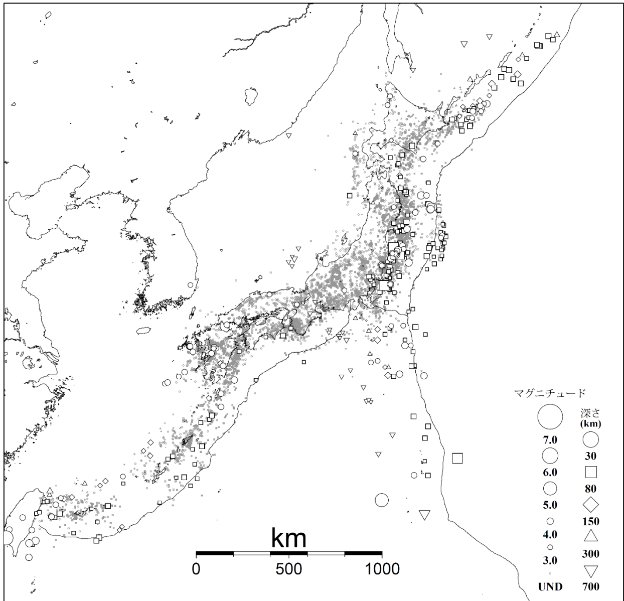
図3 気象庁が震源を決定した日本付近の平成29年2月の地震の震央分布 (M3.0以上の地震については白抜きで示す)
