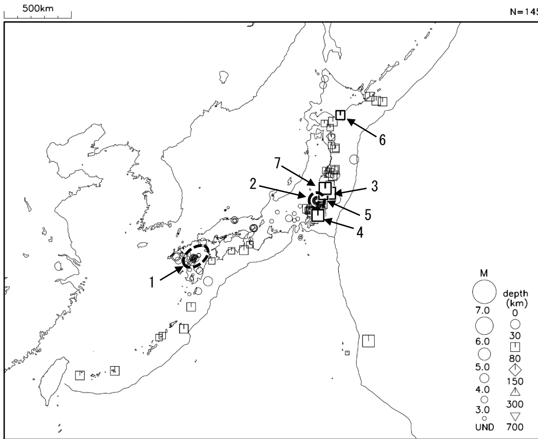
図 1 平成 29 年 2 月に震度 1 以上を観測した地震 (図中の番号は、「平成 29 年 2 月の主な地震活動」の表の番号に対応する主な地震)
