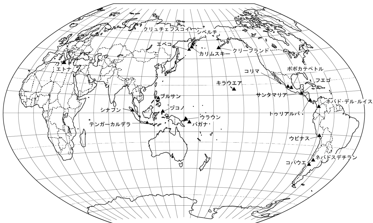
図 平成 28 年（2016 年）10 月に噴火した主な火山（日本を除く）*
