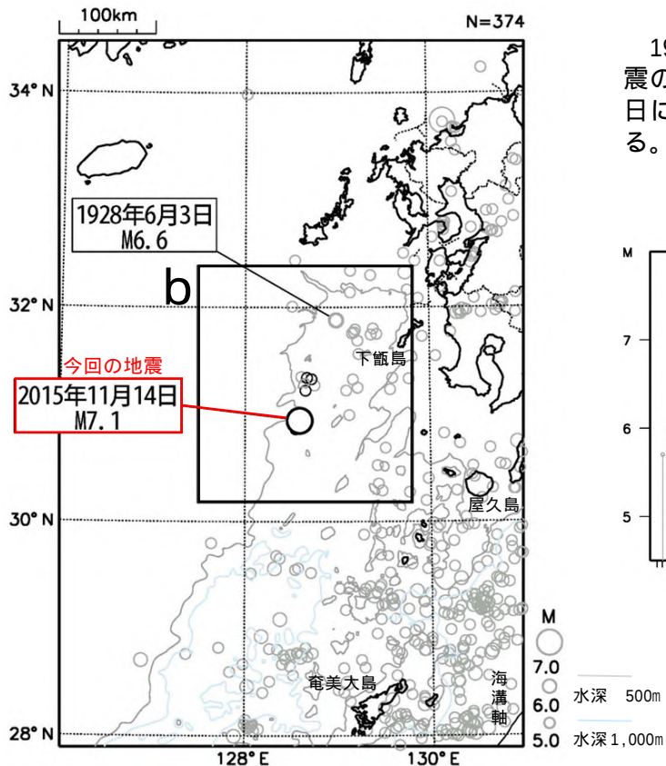
図 2 - 5 震央分布図 （1923 年 1 月 1 日～2015 年 11 月 30 日、 深さ 0 ～ 90km、M 5.0）
