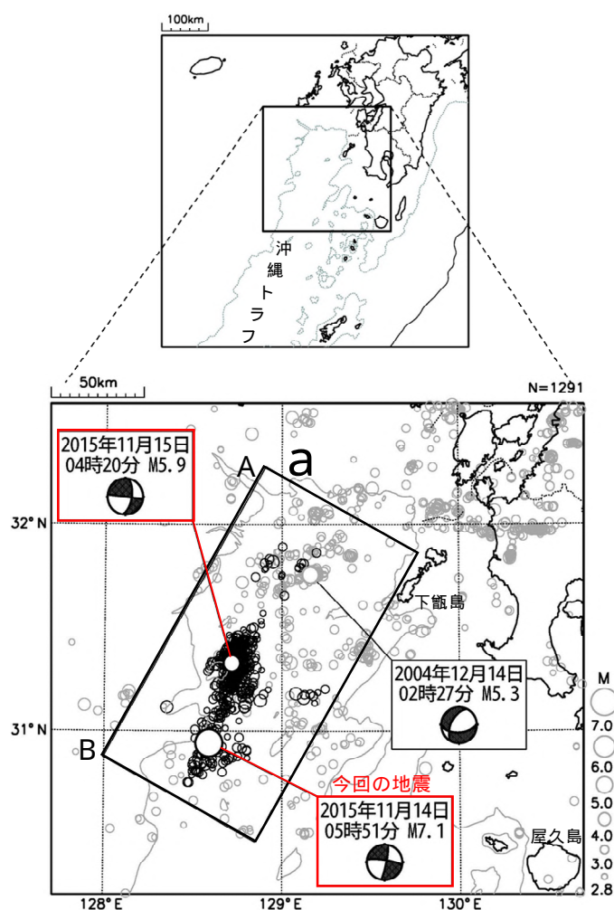
図 2 - 1 震央分布図 (1997 年 10 月 1 日 ~ 2015 年 11 月 30 日、 深さ 0 ~ 30km、M 2.8) 2015 年 11 月の地震を濃く表示 図中の発震機構は CMT 解 図中の細線は水深 500m を示す
