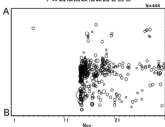
図 2 - 3 領域 a 内の時空間分布図（A - B 投影、 2015 年 11 月 1 日 ~ 30 日）
