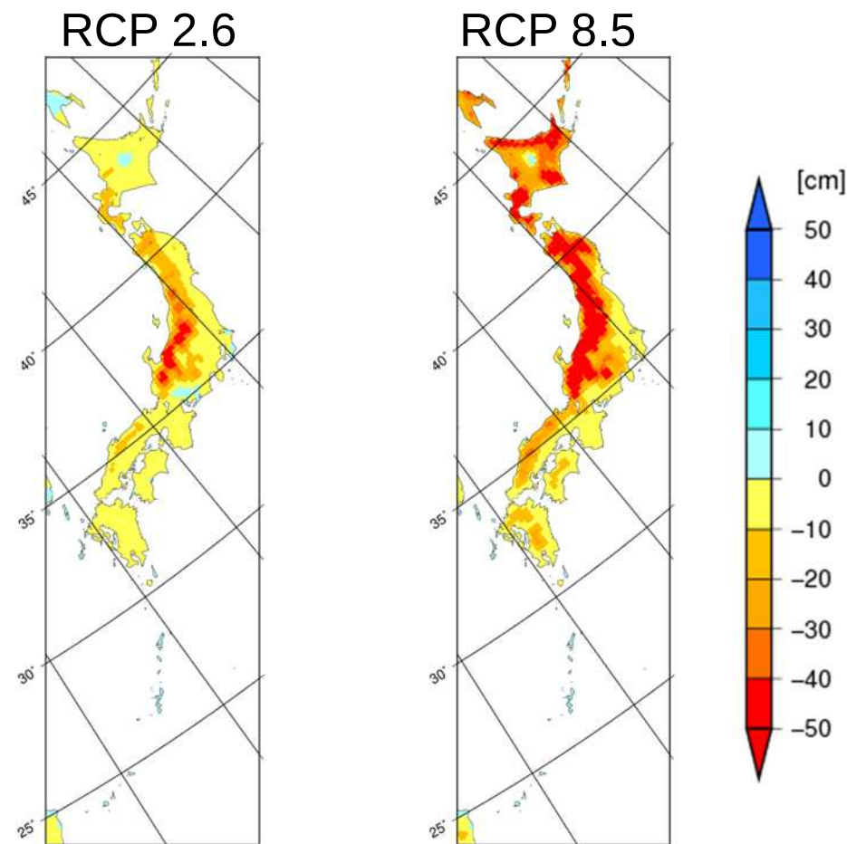
年最深積雪の変化の分布 (SST1, YSケースの例示)
