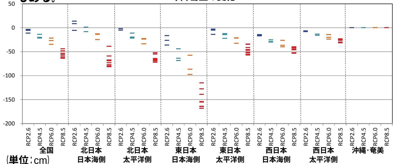
年降雪量の変化
