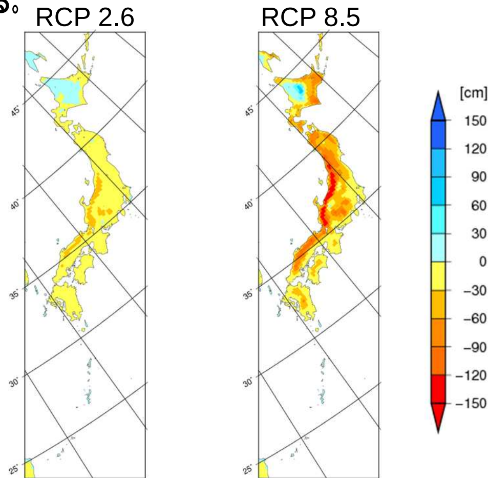
年降雪量の変化の分布 (SST1, YSケースの例示)
