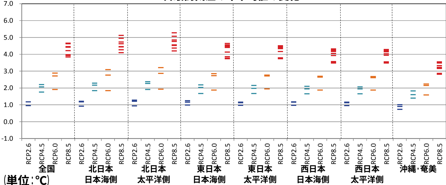
日最高気温の年平均値の変化
