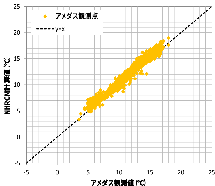
年平均気温 (20年平均)
