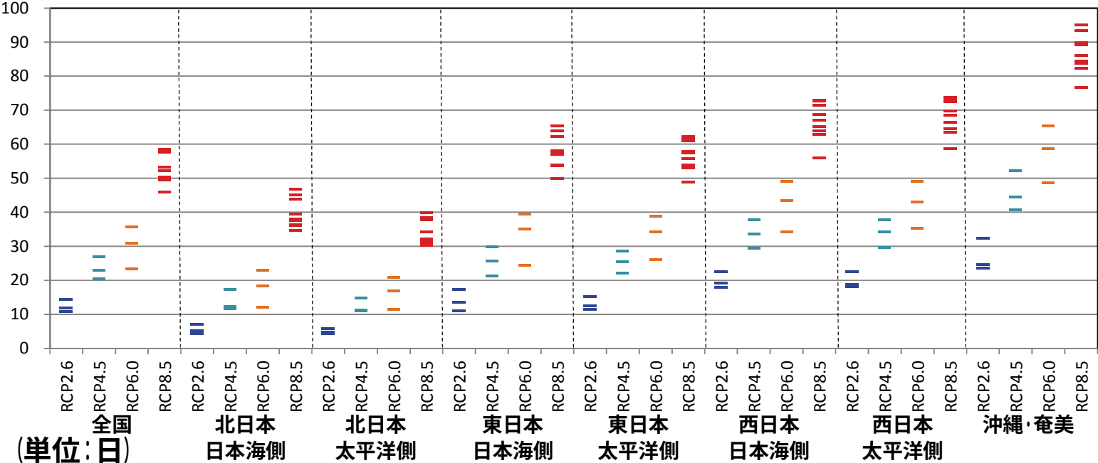
真夏日の年間日数の変化
