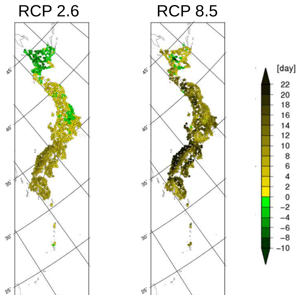
無降水日の年間日数の変化の分布 (SST1, YSケースの例示)
