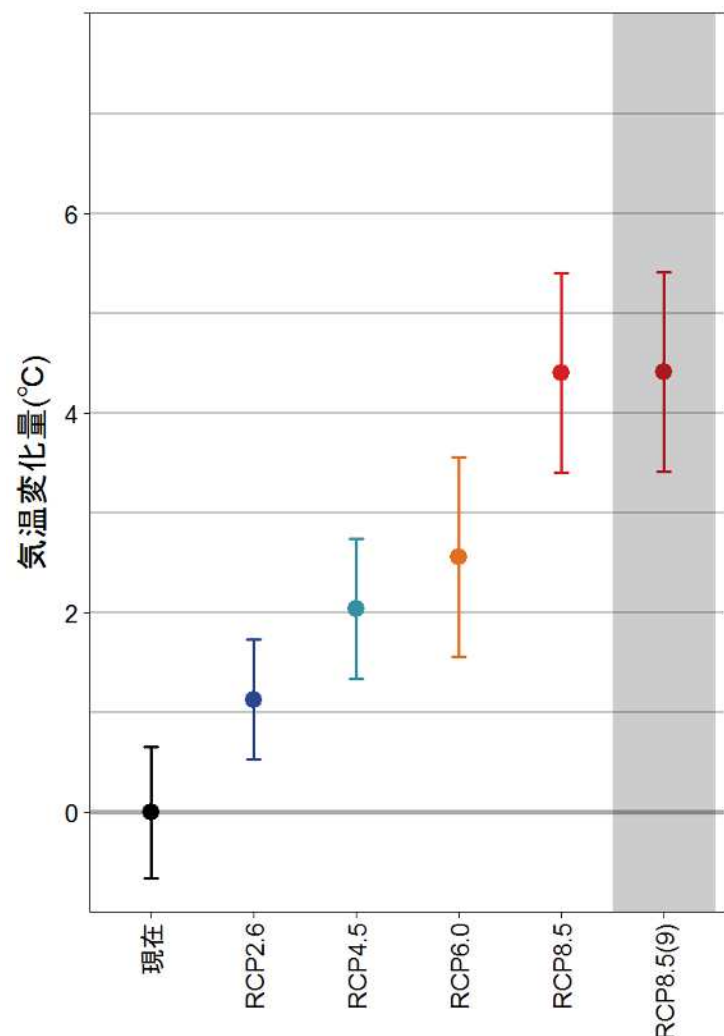
年平均気温の不確実性幅：全国
