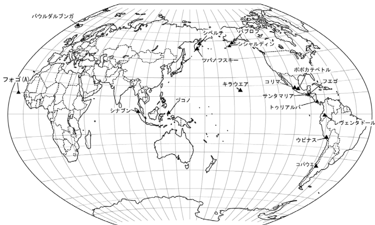
図 平成 26 年（2014 年）11 月に噴火した主な火山（日本を除く）*
