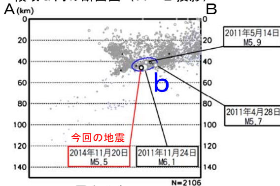
震央分布図
