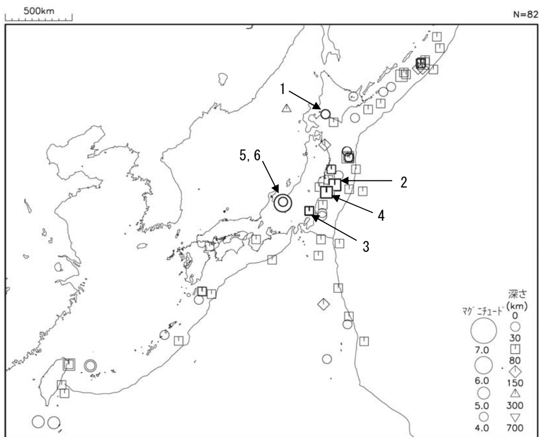
図2 平成26年11月に発生したM4.0以上の地震 (図中の番号は、「平成26年11月の主な地震活動」の表の番号に対応する主な地震)
