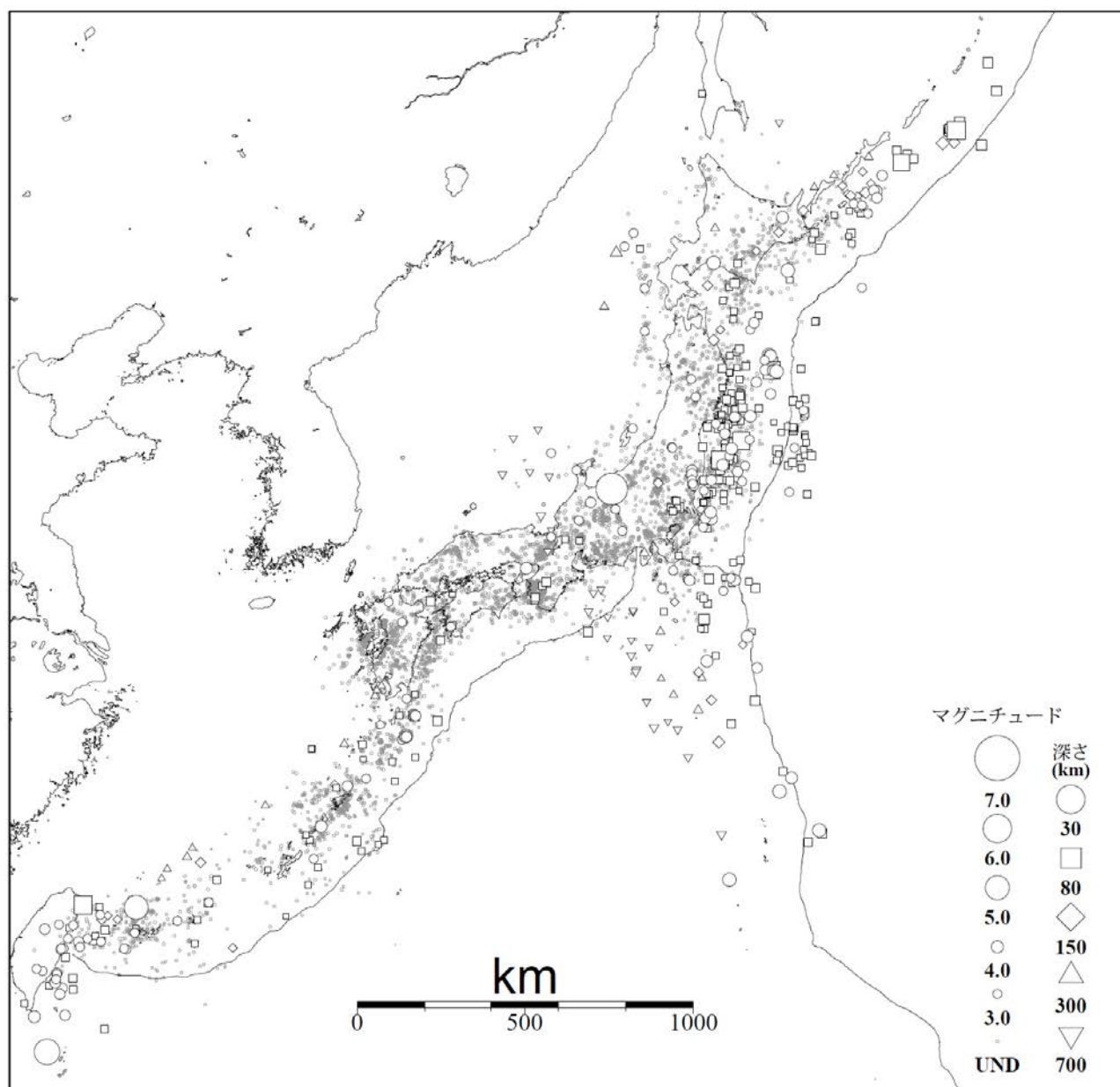
図3 気象庁が震源を決定した日本付近の平成26年11月の地震の震央分布 (M3.0以上の地震については白抜きで示す)
