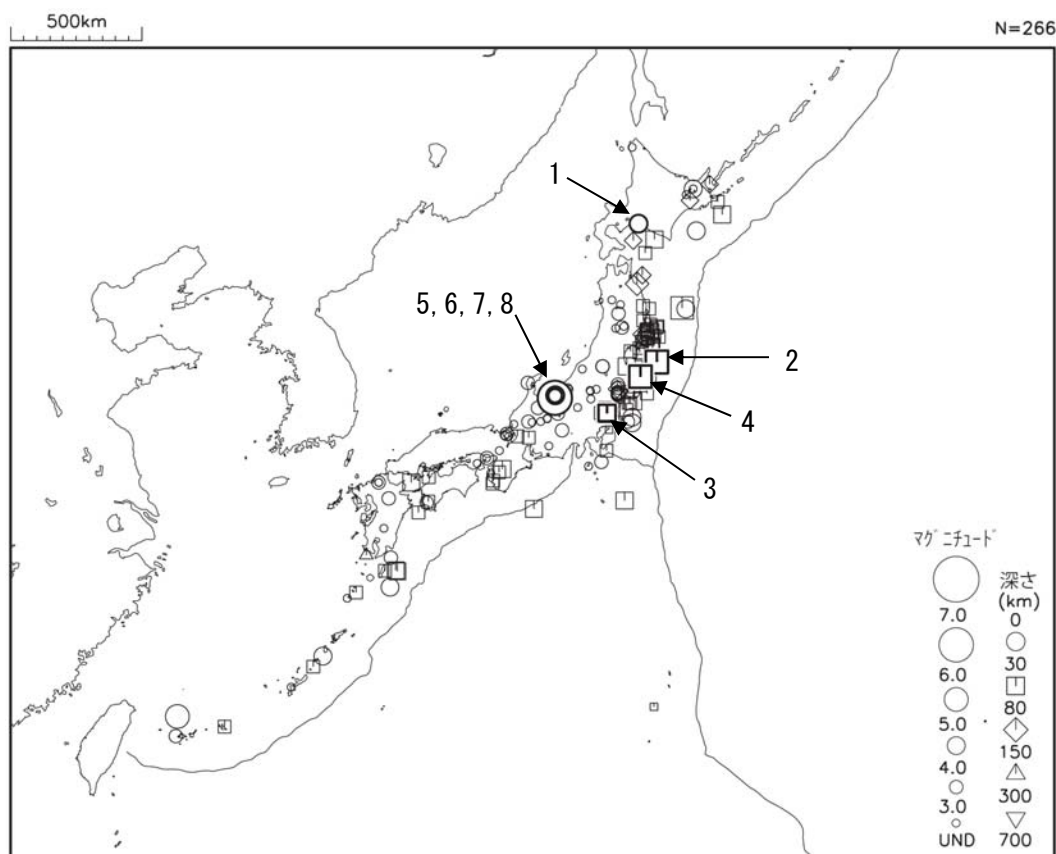
図1 平成26年11月に震度1以上を観測した地震 (図中の番号は、「平成26年11月の主な地震活動」の表の番号に対応する主な地震)
