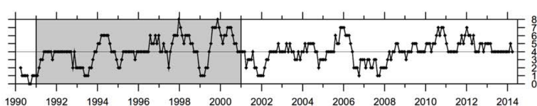
図3 東海地域の地震活動指数の推移
