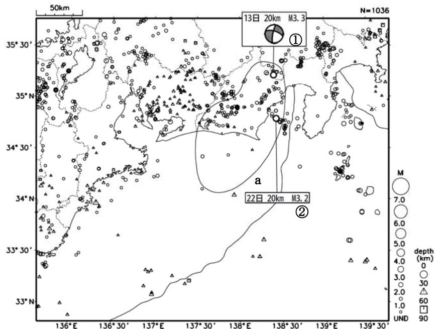
図1 震央分布図（2014年6月1日～30日：深さ0～90km、Mすべて。図中の領域aは東海地震の想定震源域。）
