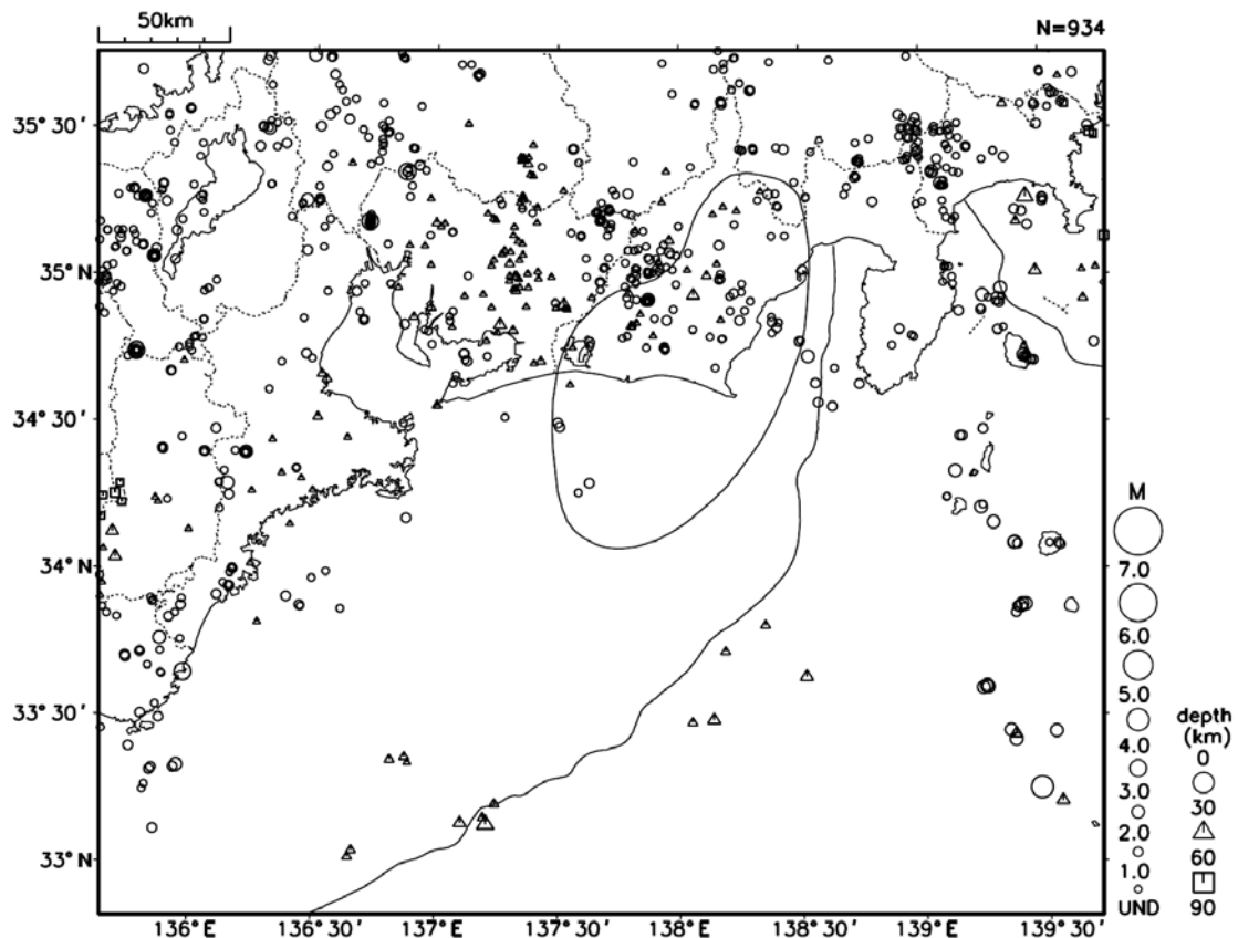
図1 震央分布図(2013年12月1日～31日: 深さ0～90km、Mすべて。図中のナス型の領域は東海地震の想定震源域。)
